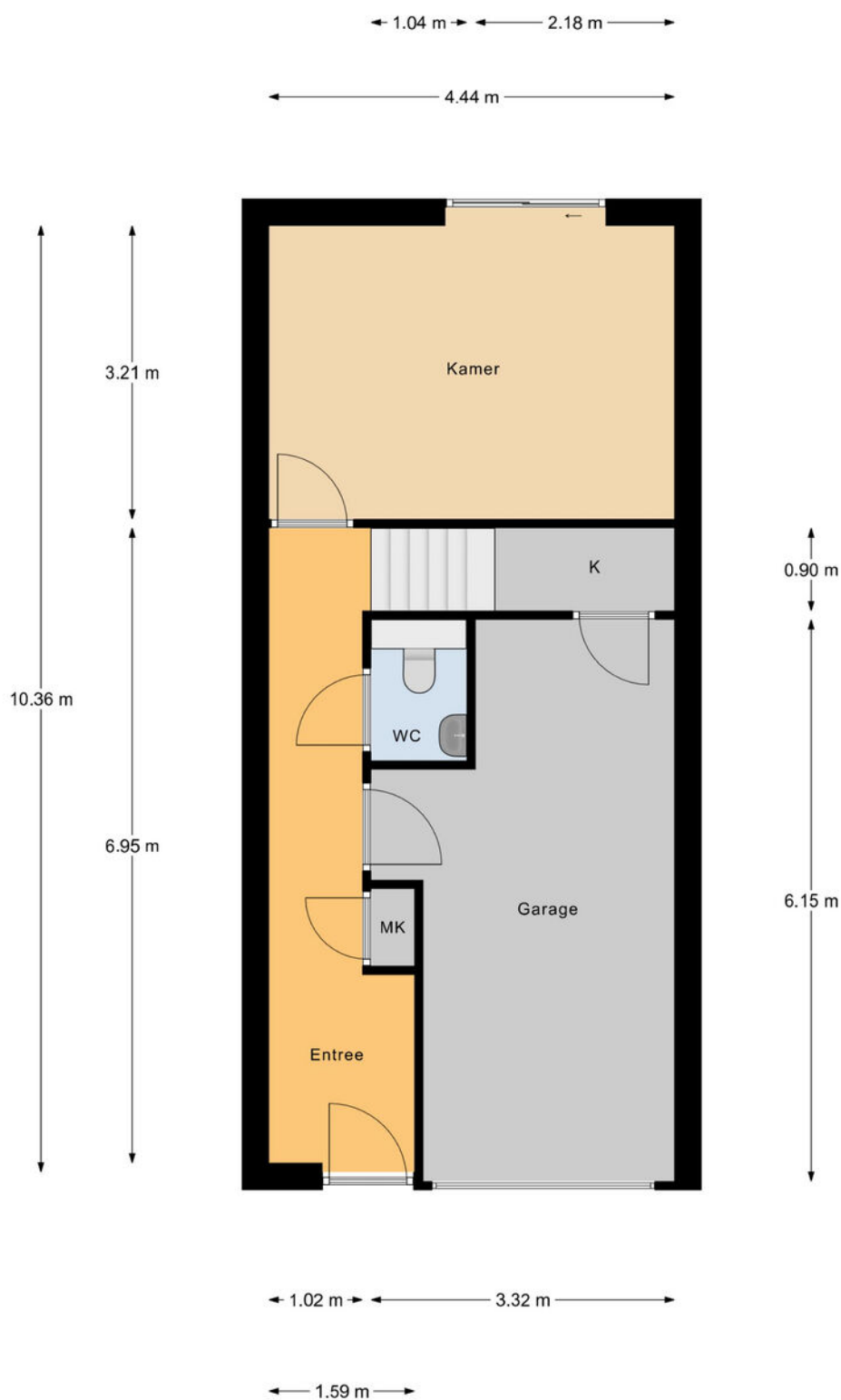
Begane Grond
