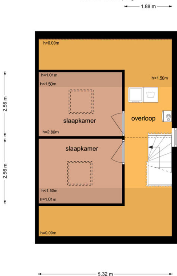
De Vlierbes 42 - Doetinchem Tweede Verdieping
