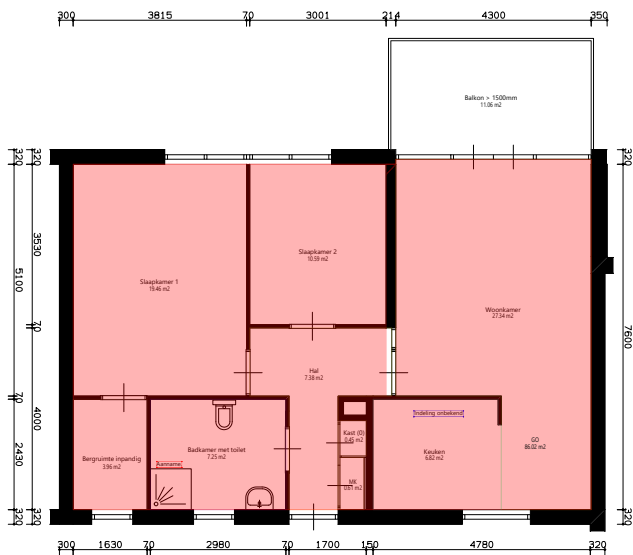
Verdieping_1e
