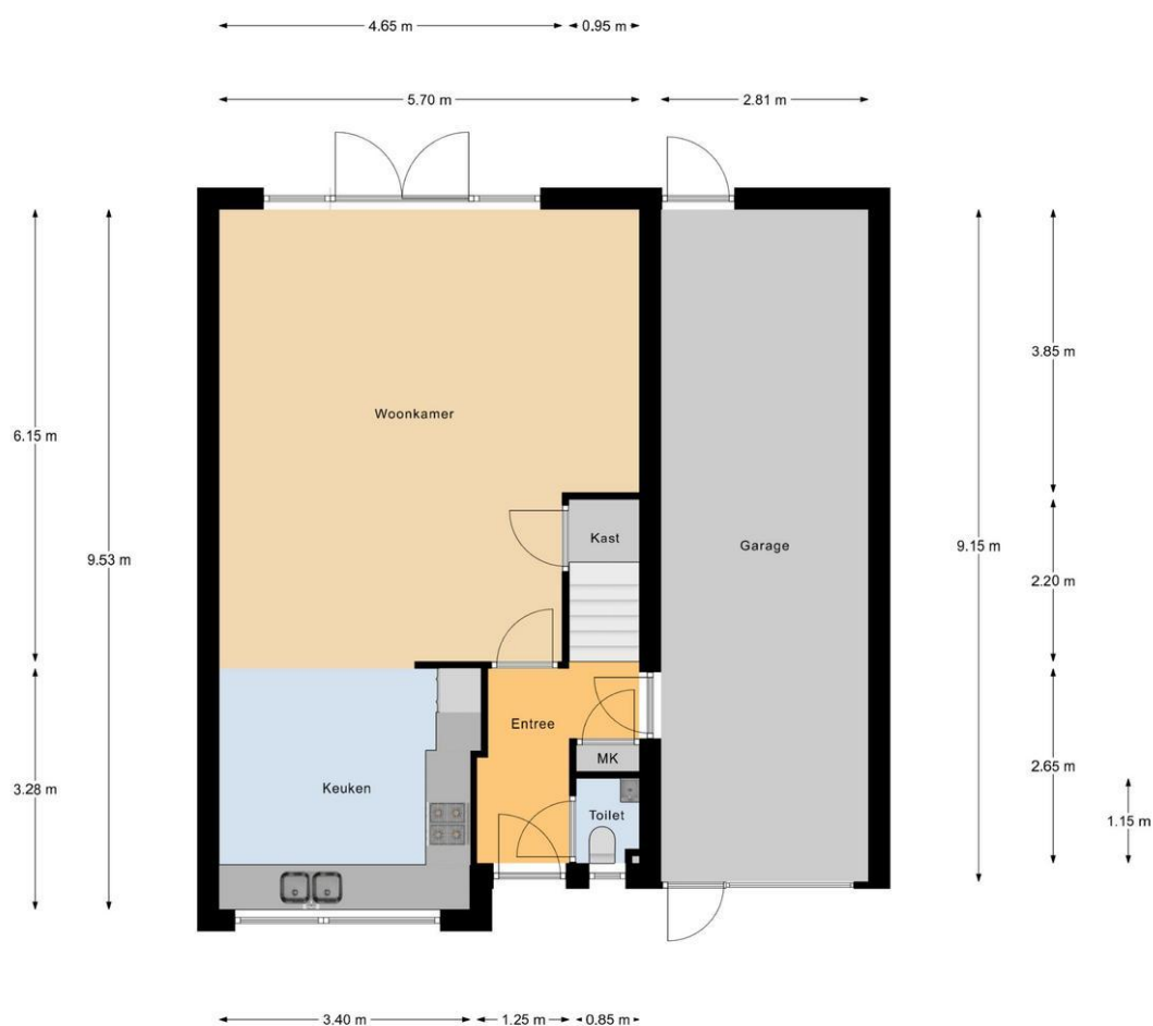
Begane Grond
