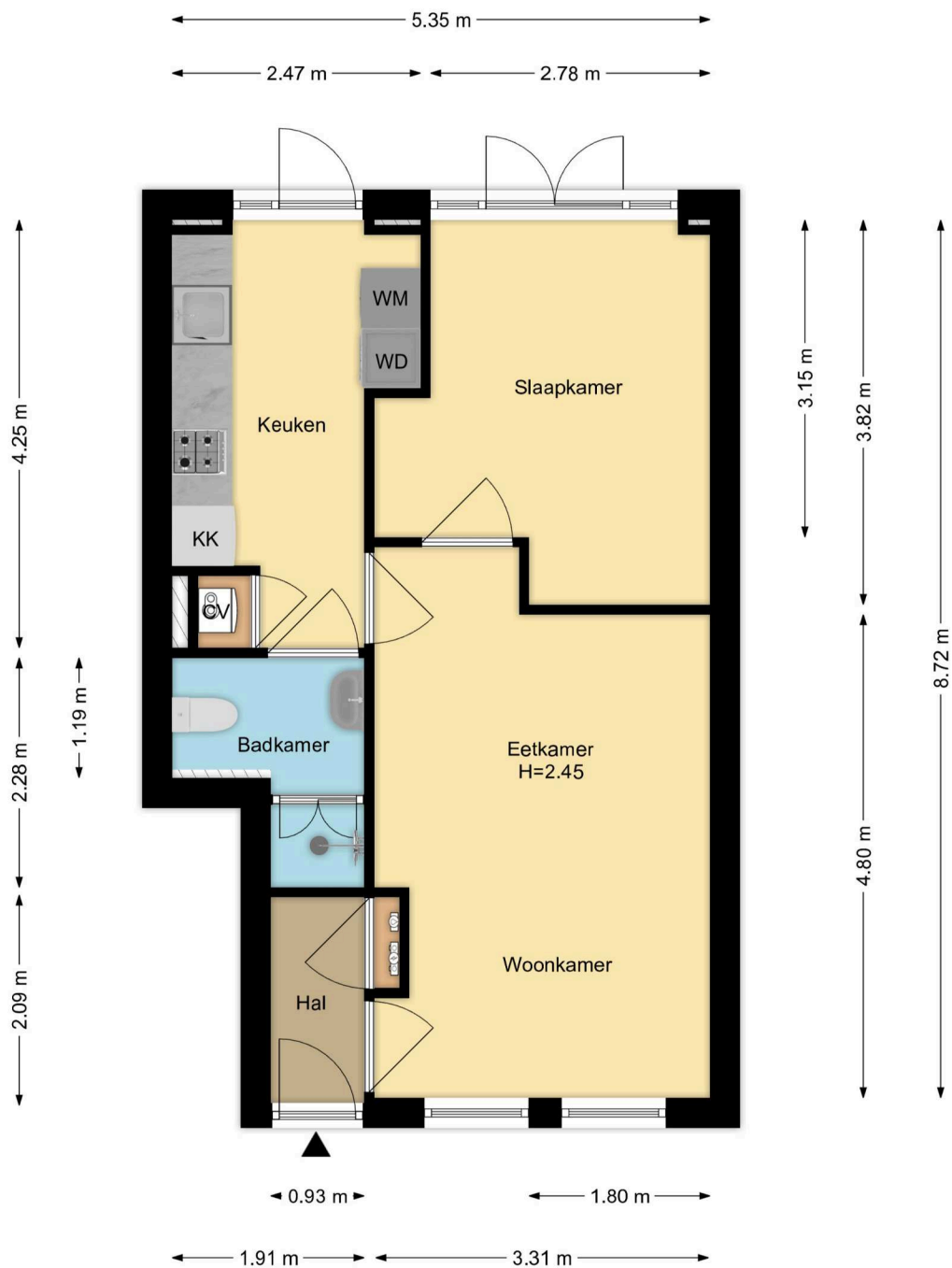
Begane Grond Bakkerstraat 74 Zwart, Haarlem R.M. Vastgoedpresentatie| Aan deze plattegrond kunnen geen rechten worden ontleend
