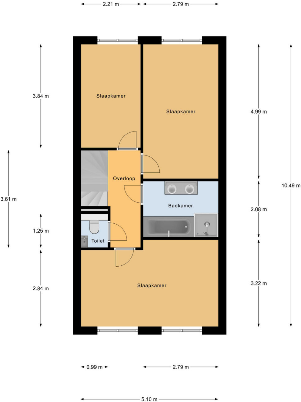
1e Verdieping
