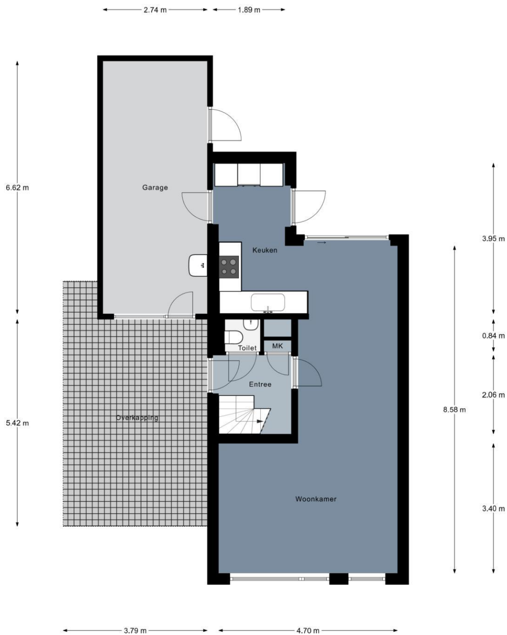
Begane Grond
