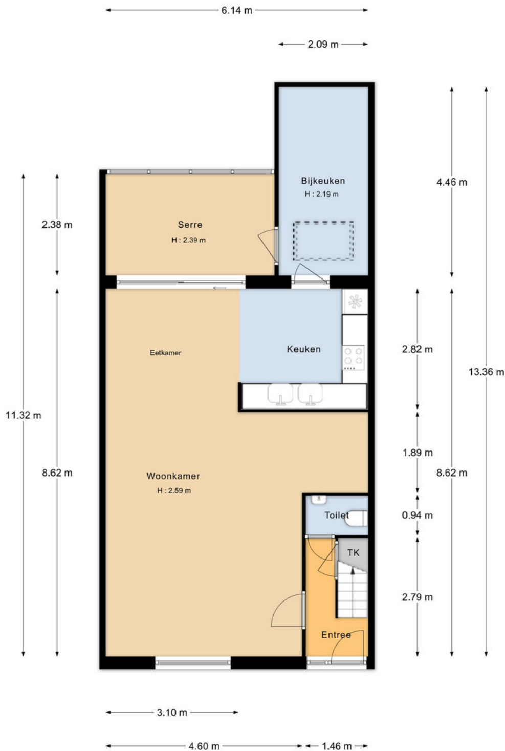
Begane grond
