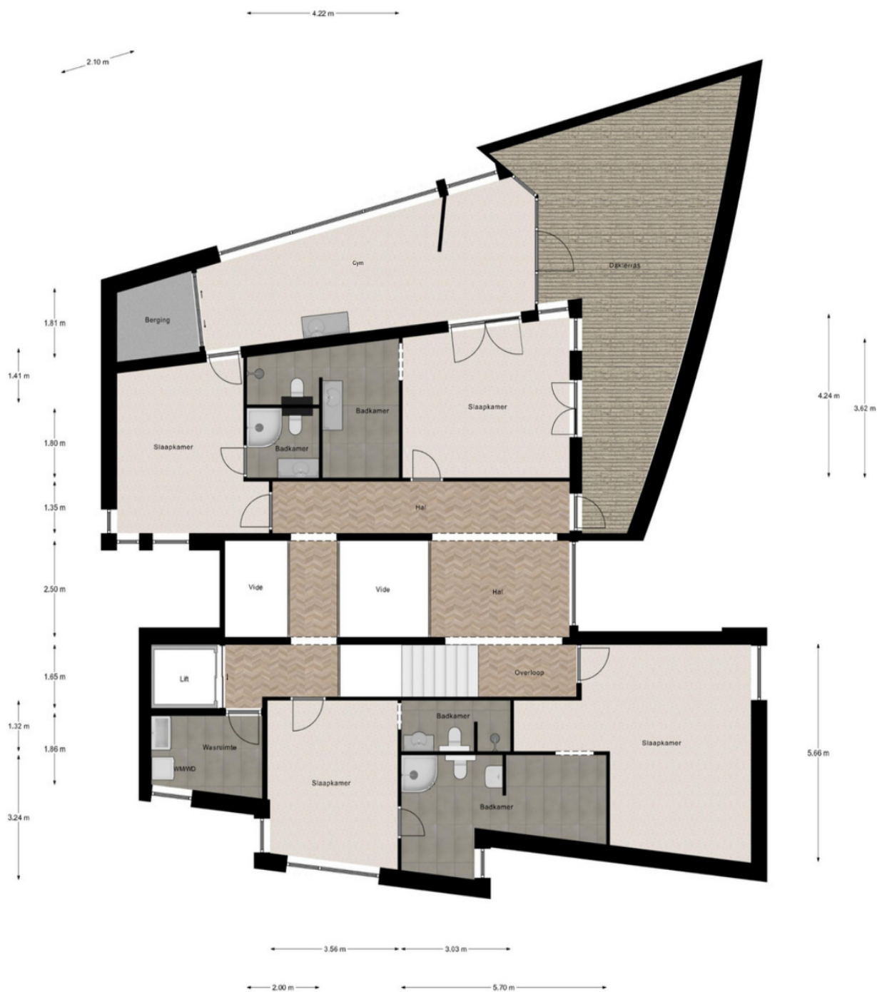
Eerste Verdieping
