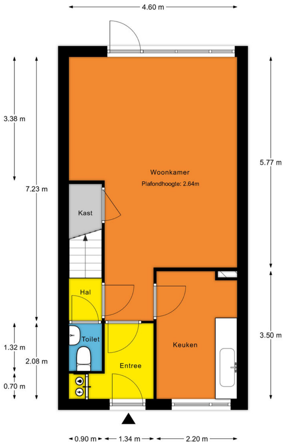
Begane grond
