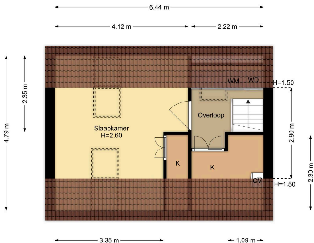
2e Verdieping Brahmslaan 29, Heemstede R.M. Vastgoedpresentatie | Aan deze plattegrond kunnen geen rechten worden ontleend
