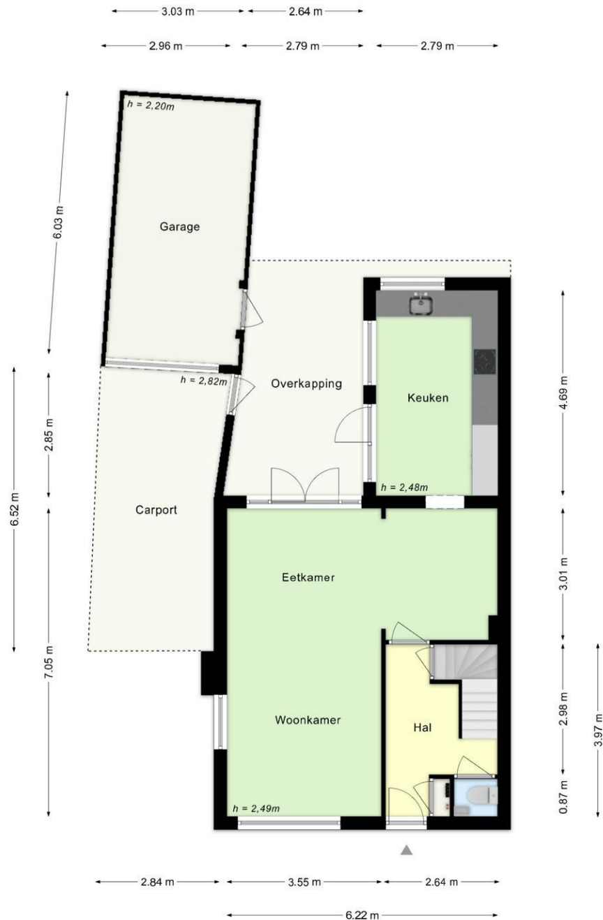
De Gyselaar 5 Amstenrade - Begane grond
