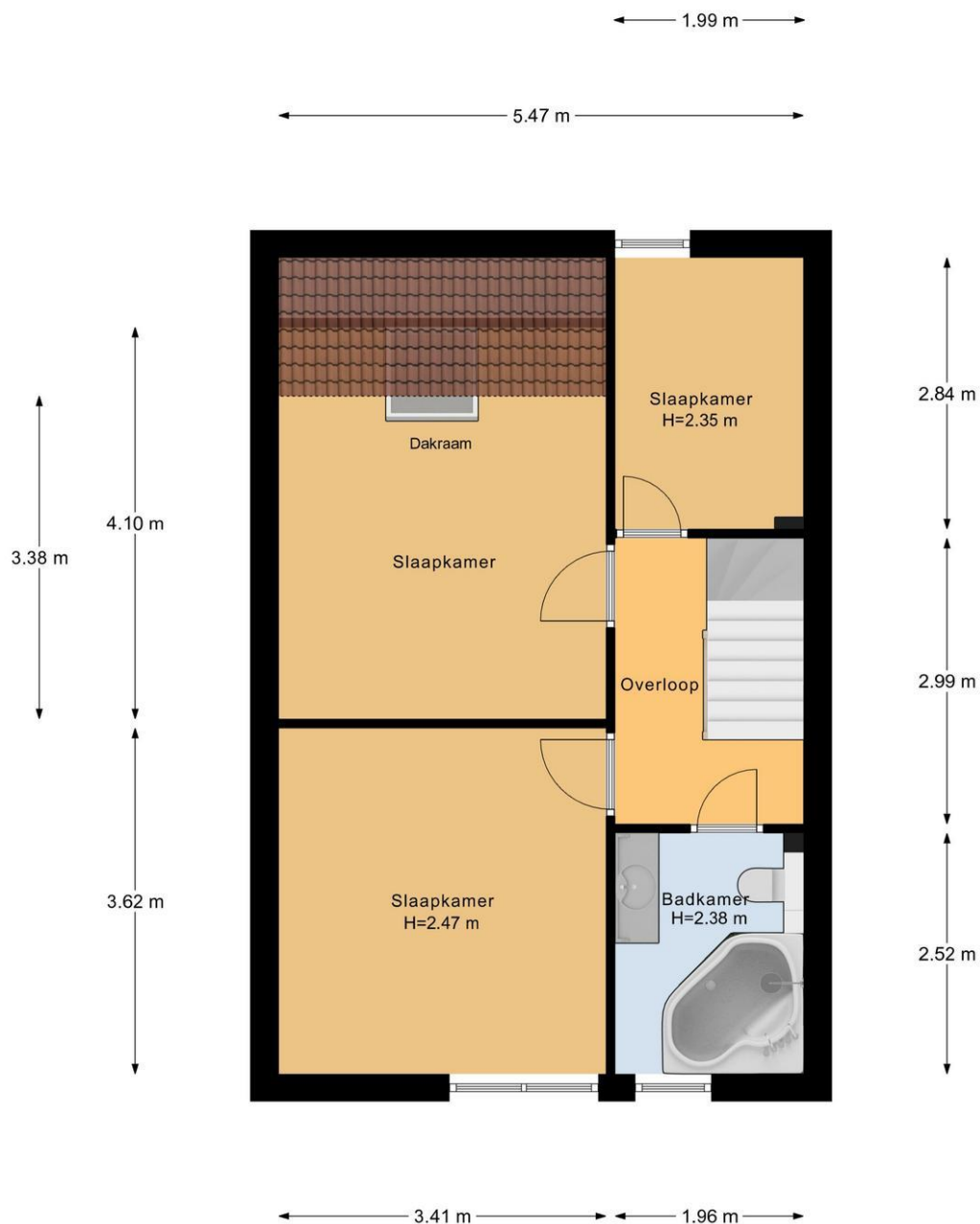
1e Verdieping
