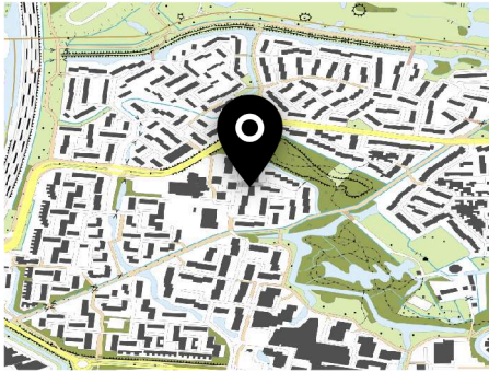
Kadastrale kaart
