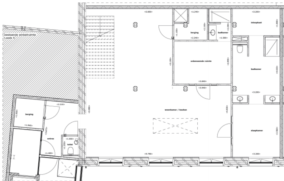
Plattegrond verdieping 01 1:50
