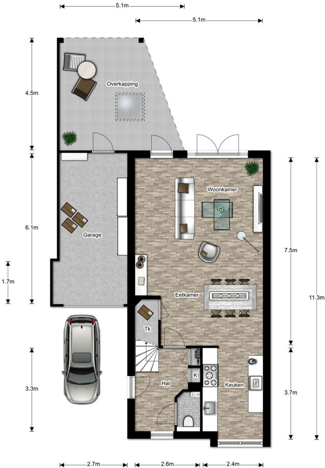
Begane grond, Antonius van Lieropstraat 29 te Heeze De plattegronden zijn ter indicatie en geproduceerd voor promotionele doeleinden.
