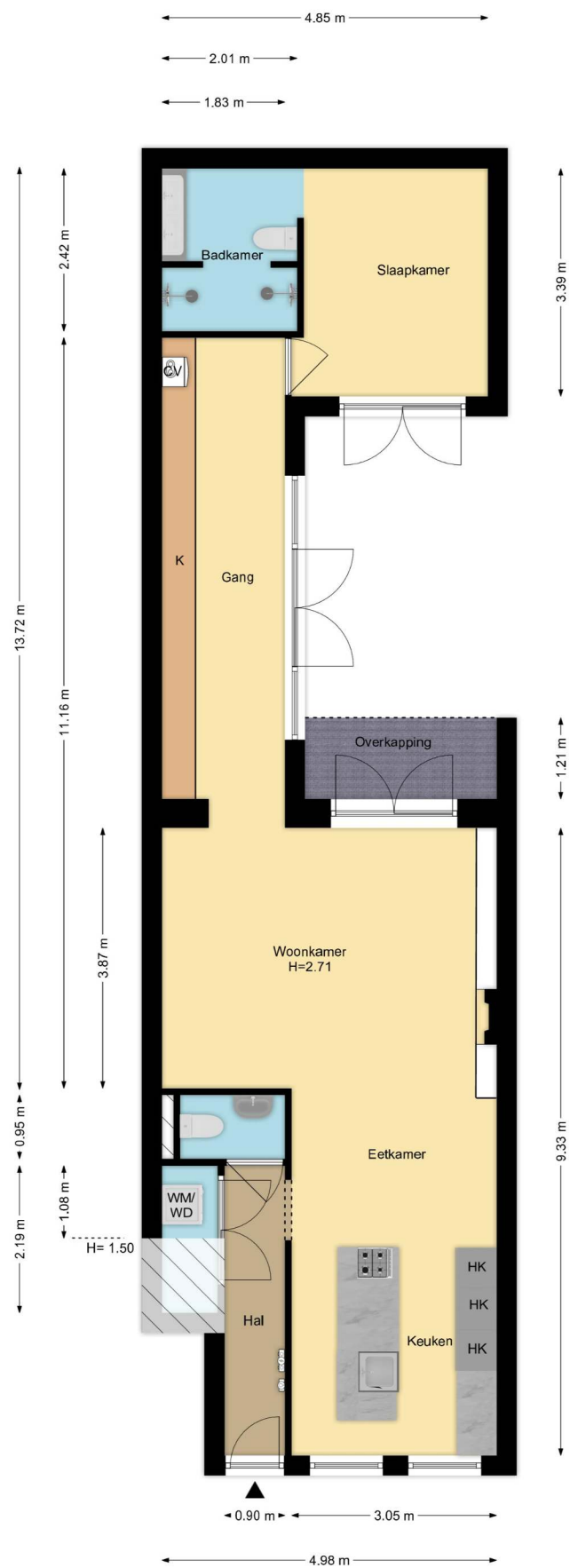
Begane Grond Vooruitgangstraat 139, Haarlem R.M. Vastgoedpresentatie| Aan deze plattegrond kunnen geen rechten worden ontleend
