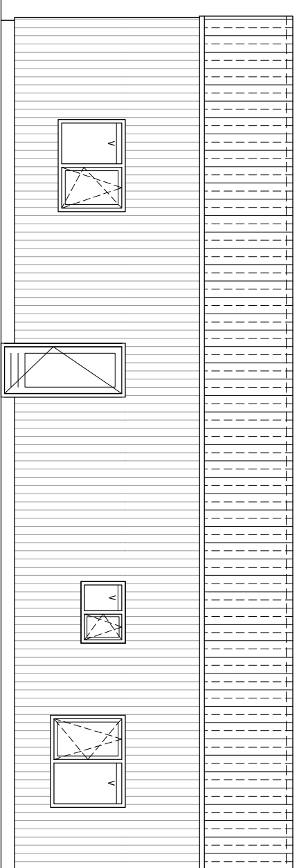
Achtergevel
