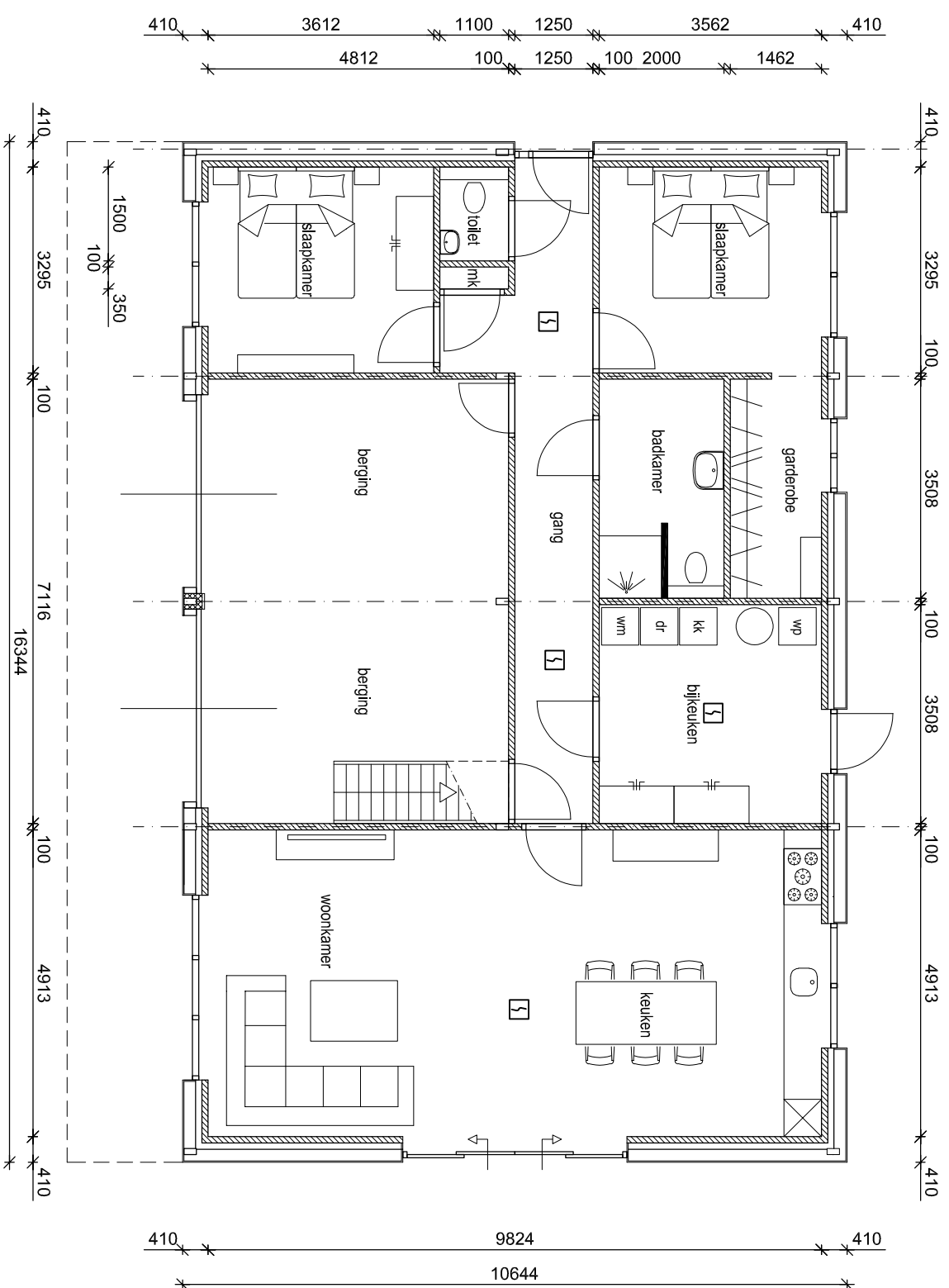
Begane grond
