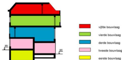
Figuur 1: Bouwlagen (Bron: NEN 2580)
