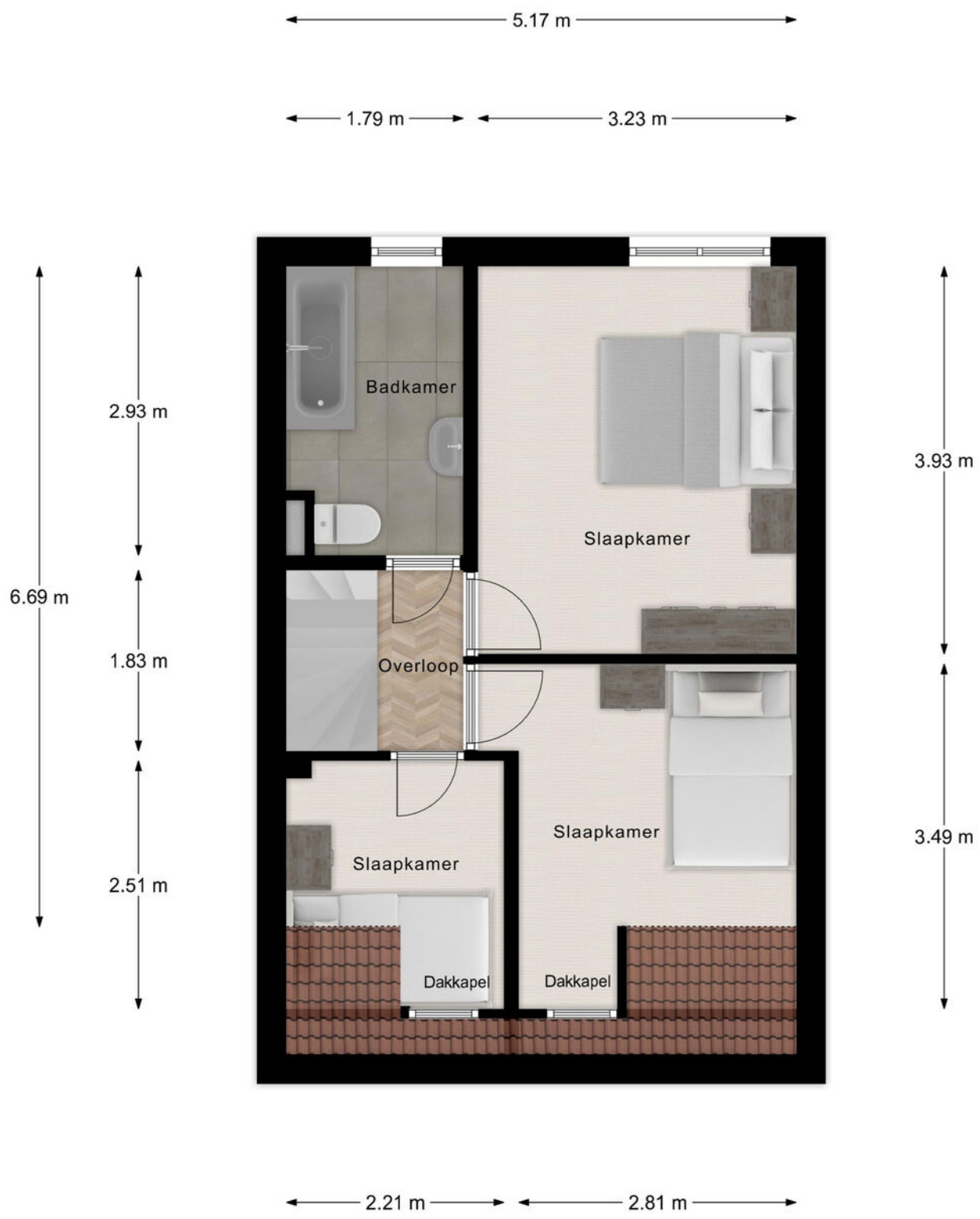
1e Verdieping
