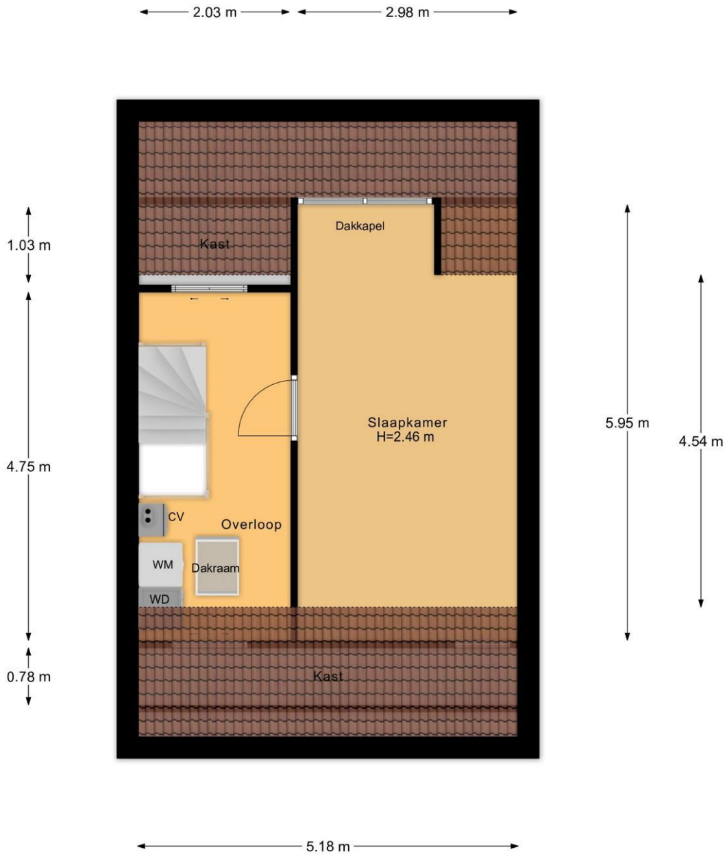
2e Verdieping
