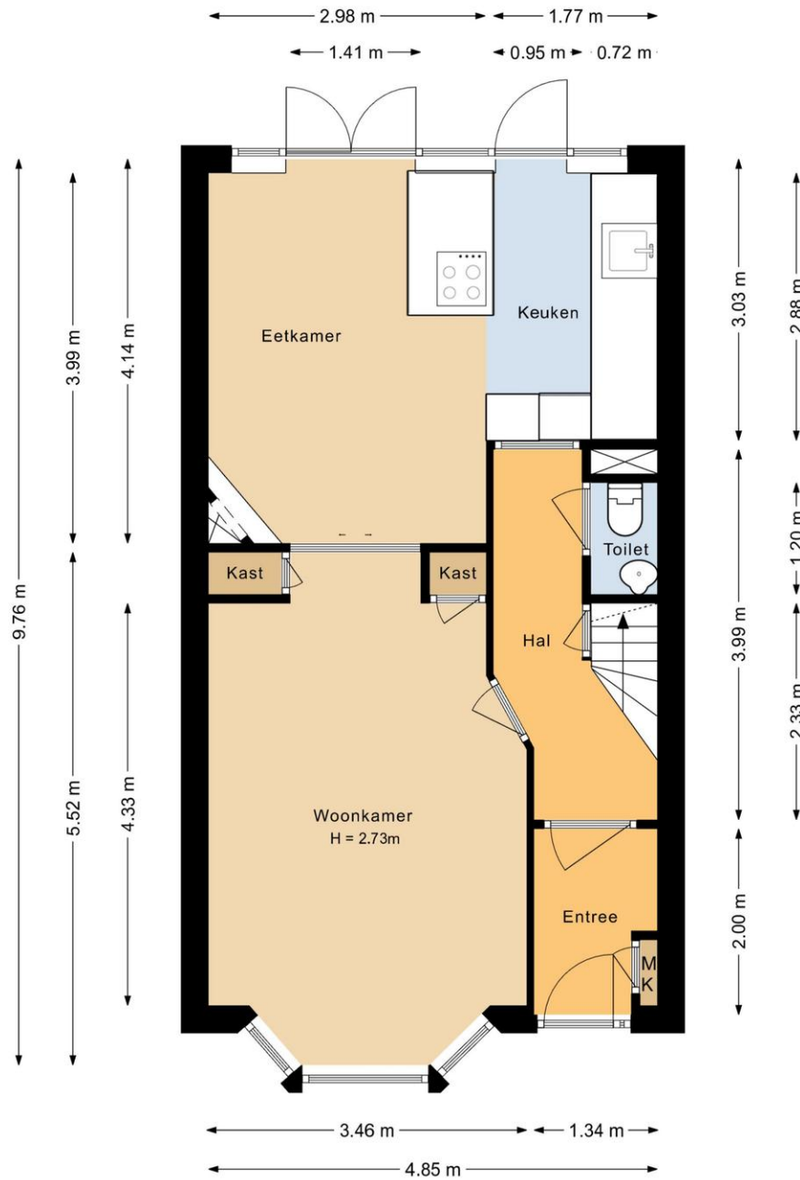
Begane grond Zonnebloemstraat 35 Haarlem
