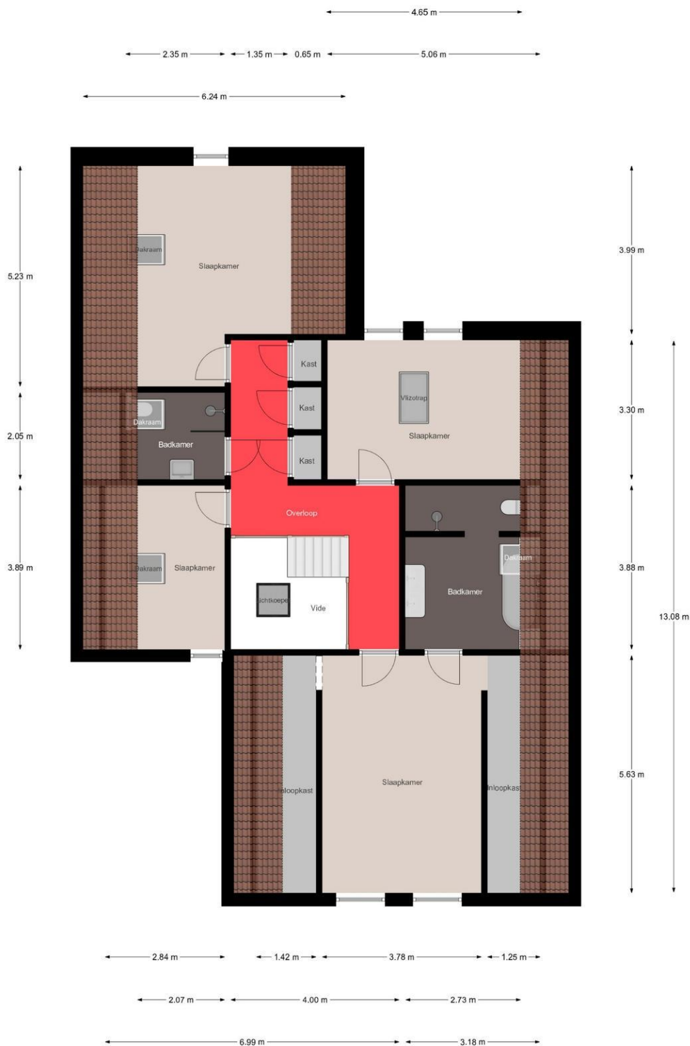
1e Verdieping
