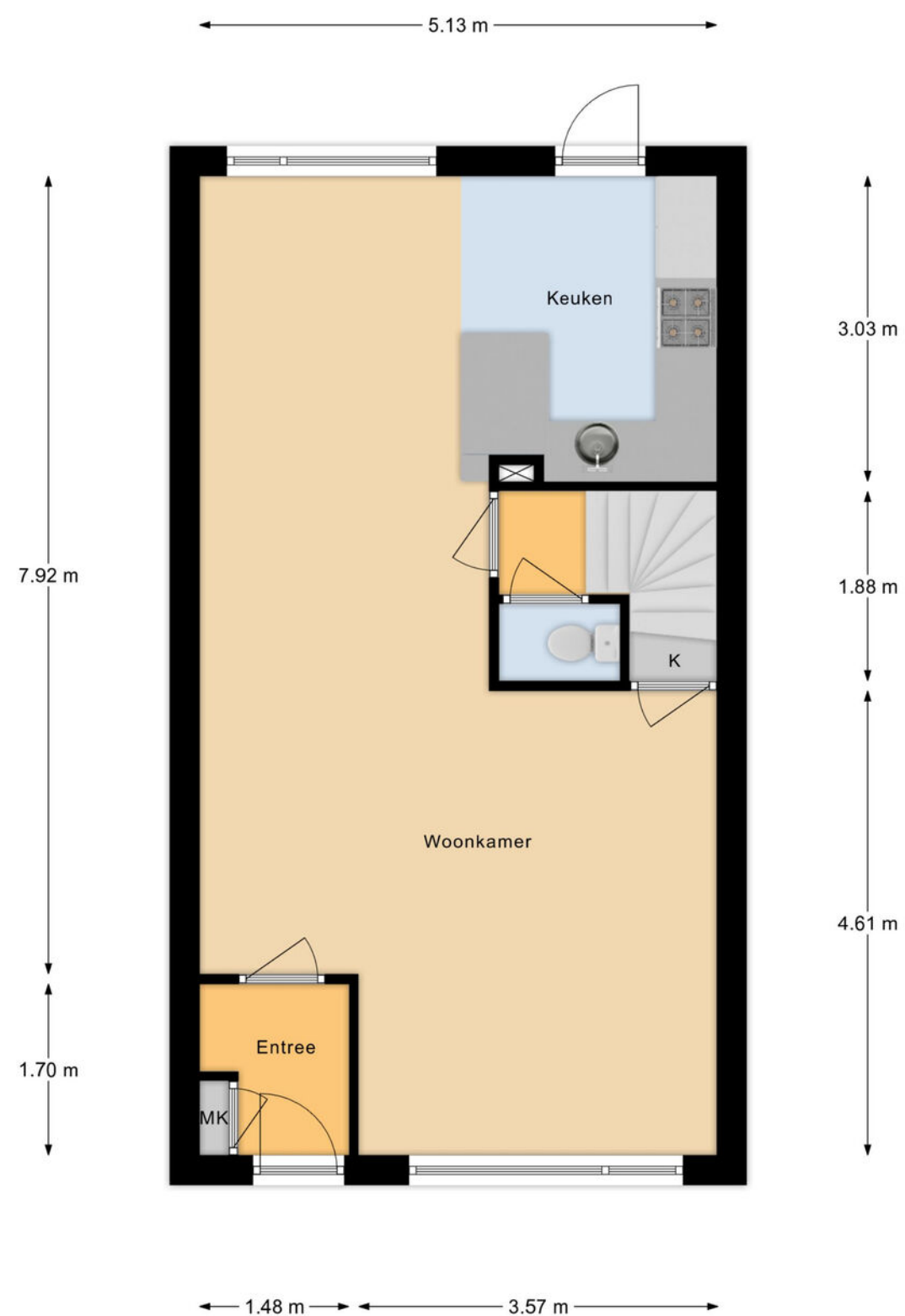
Begane Grond
