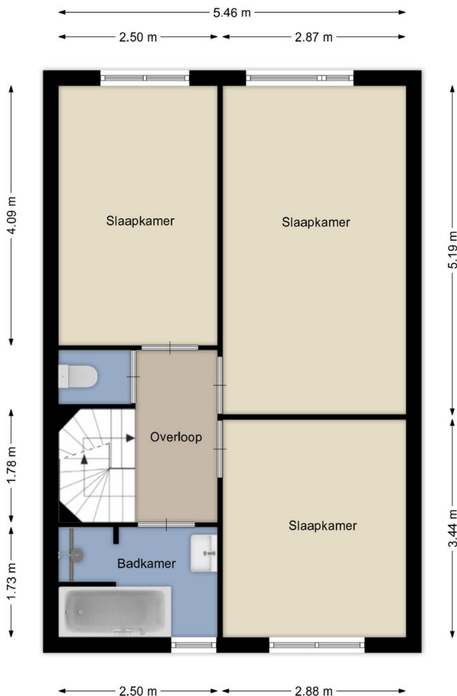
Eerste verdieping Karperborch 21, Rosmalen
