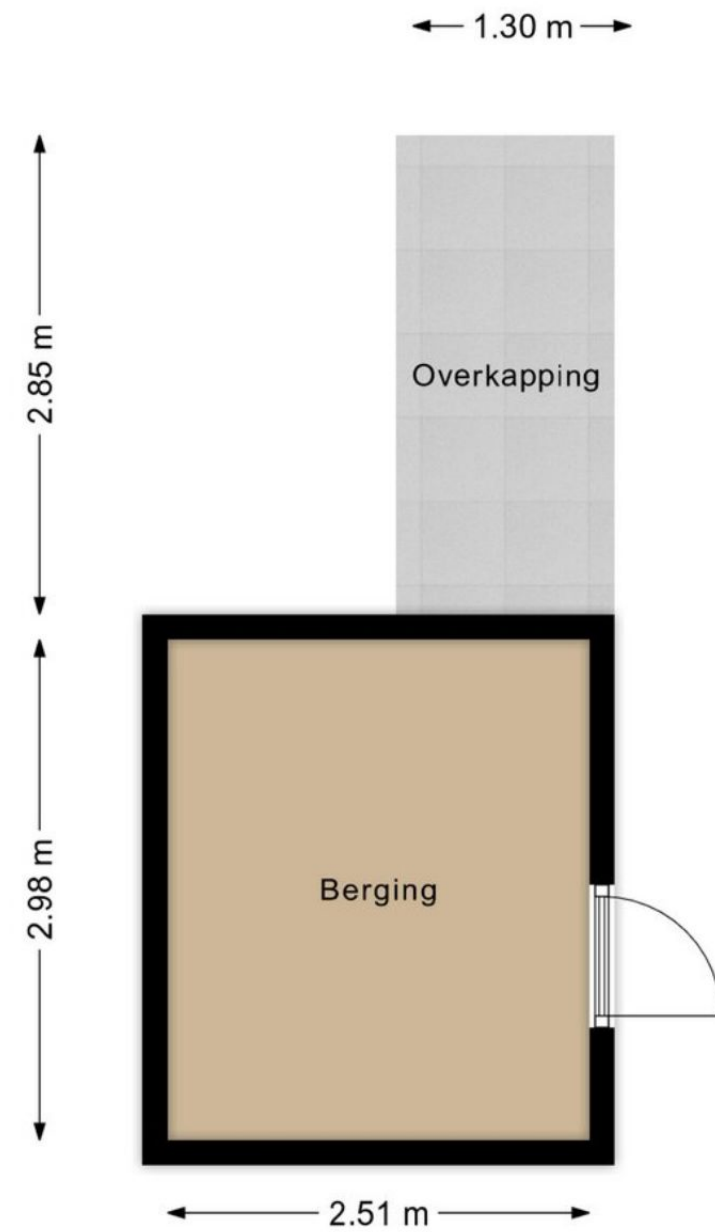
Plattegrond berging Aan deze tekening kunnen geen rechten worden ontleend.
