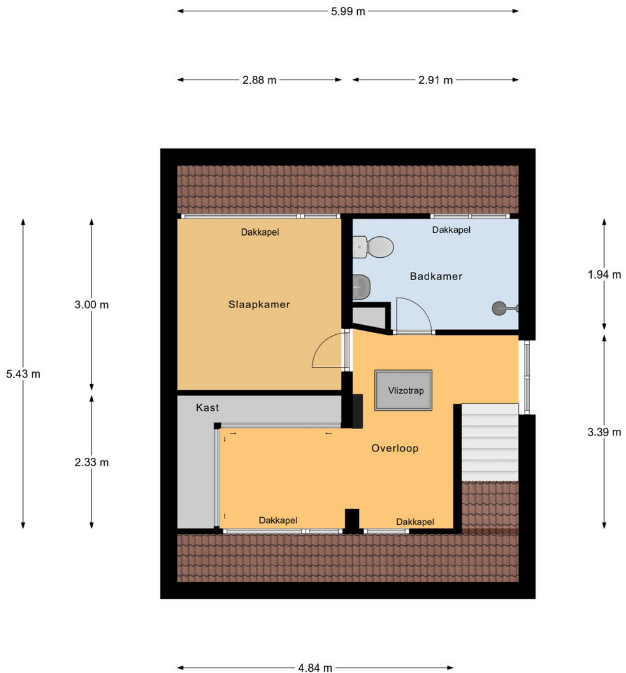
1e Verdieping
