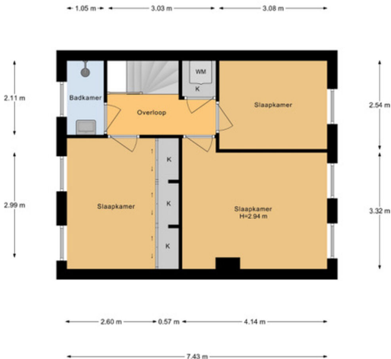
1e Verdieping
