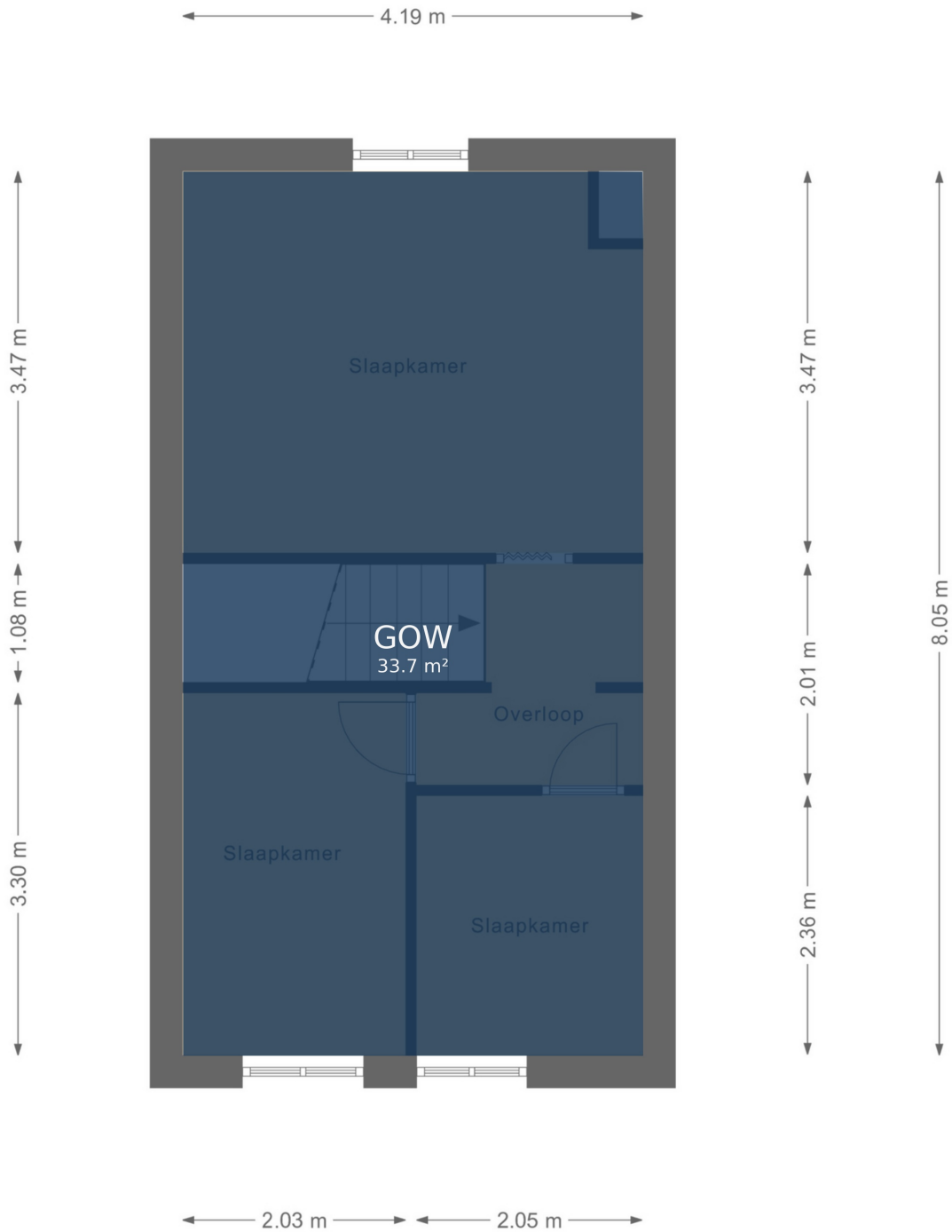
1e Verdieping
