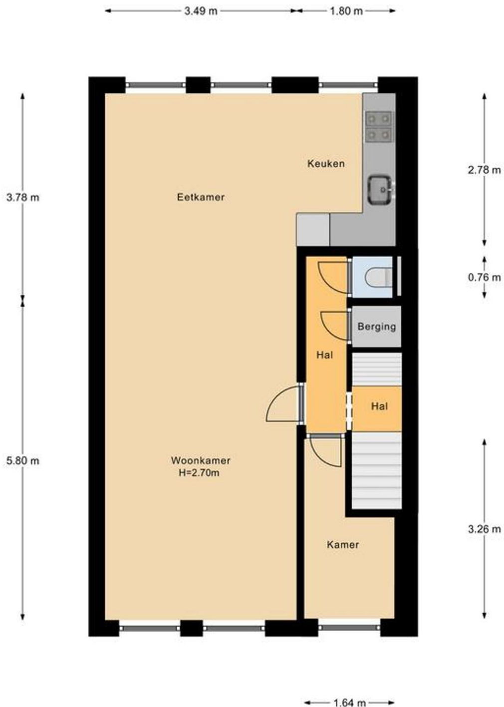
1e Verdieping
