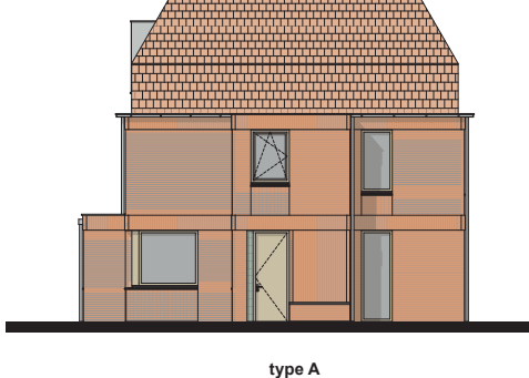
Rechtergevel
