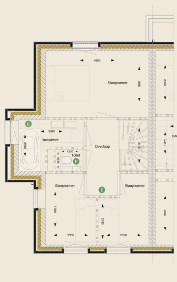
Eerste verdieping
