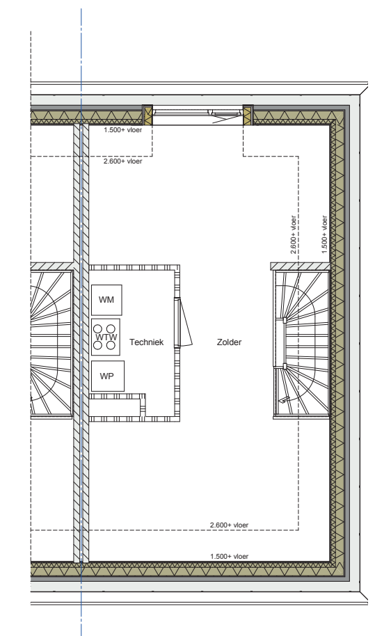
Tweede verdieping
