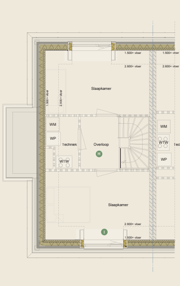
Tweede verdieping
