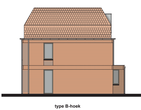
Linkergevel
