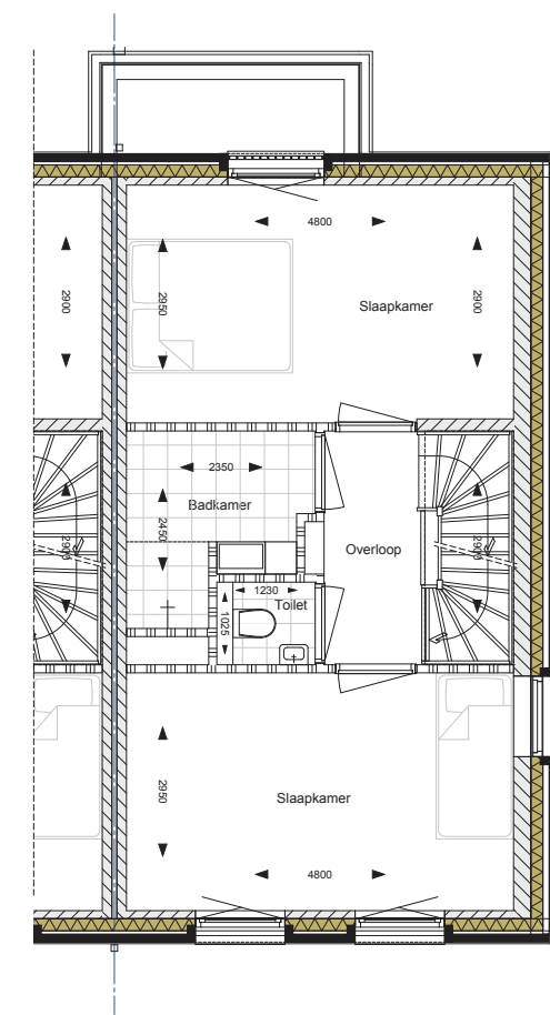
Eerste verdieping
