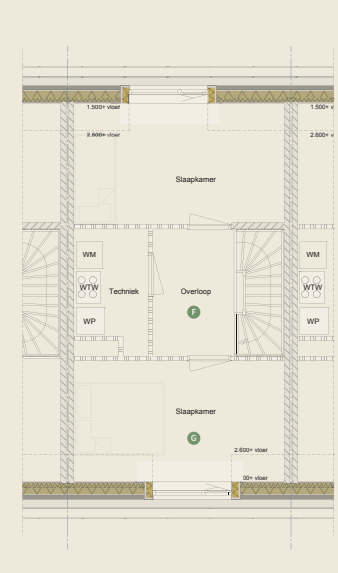
Tweede verdieping
