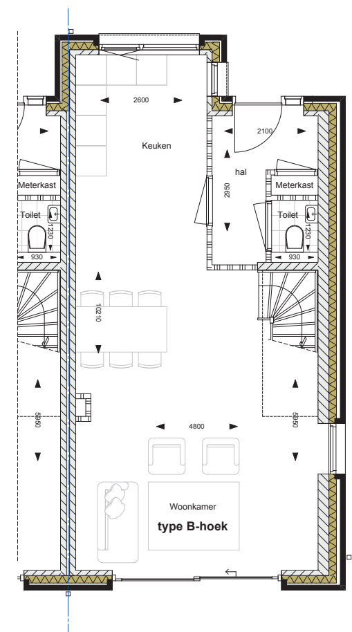
Begane grond
