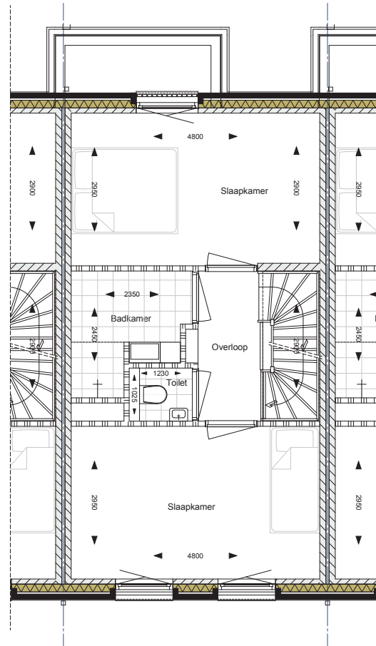
Eerste verdieping
