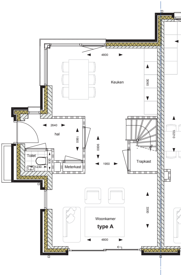
Begane grond
