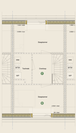
Tweede verdieping
