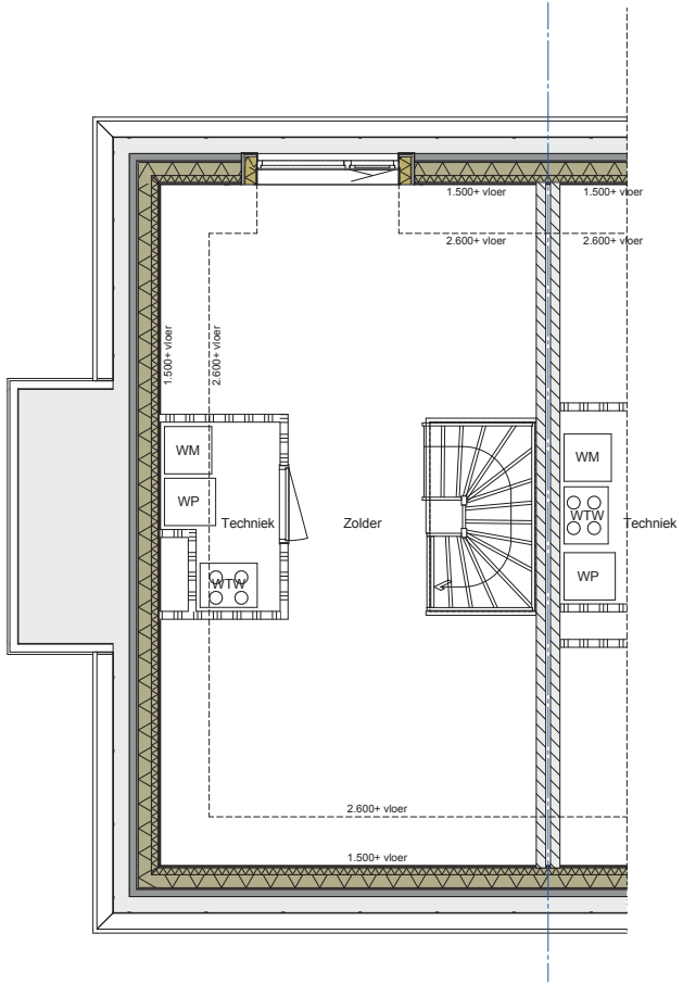
Tweede verdieping
