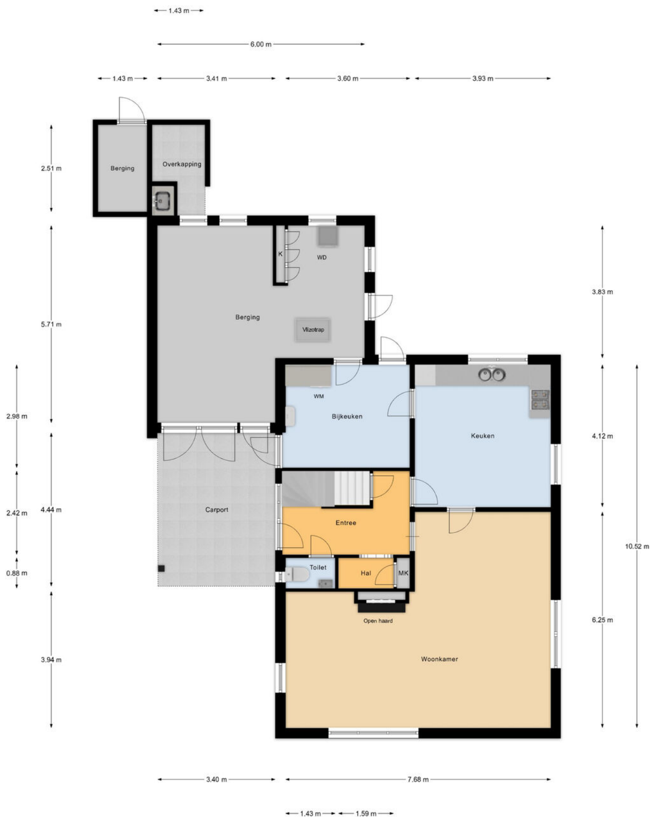
Begane Grond
