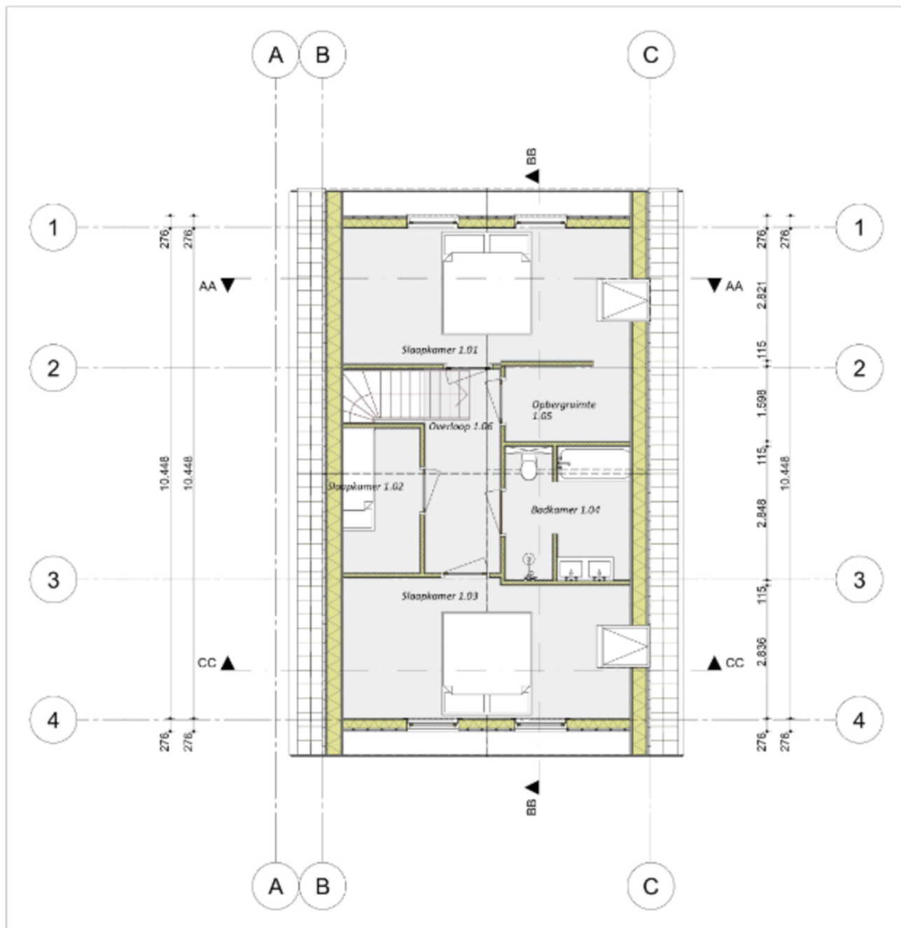
1e verdieping woonhuis
