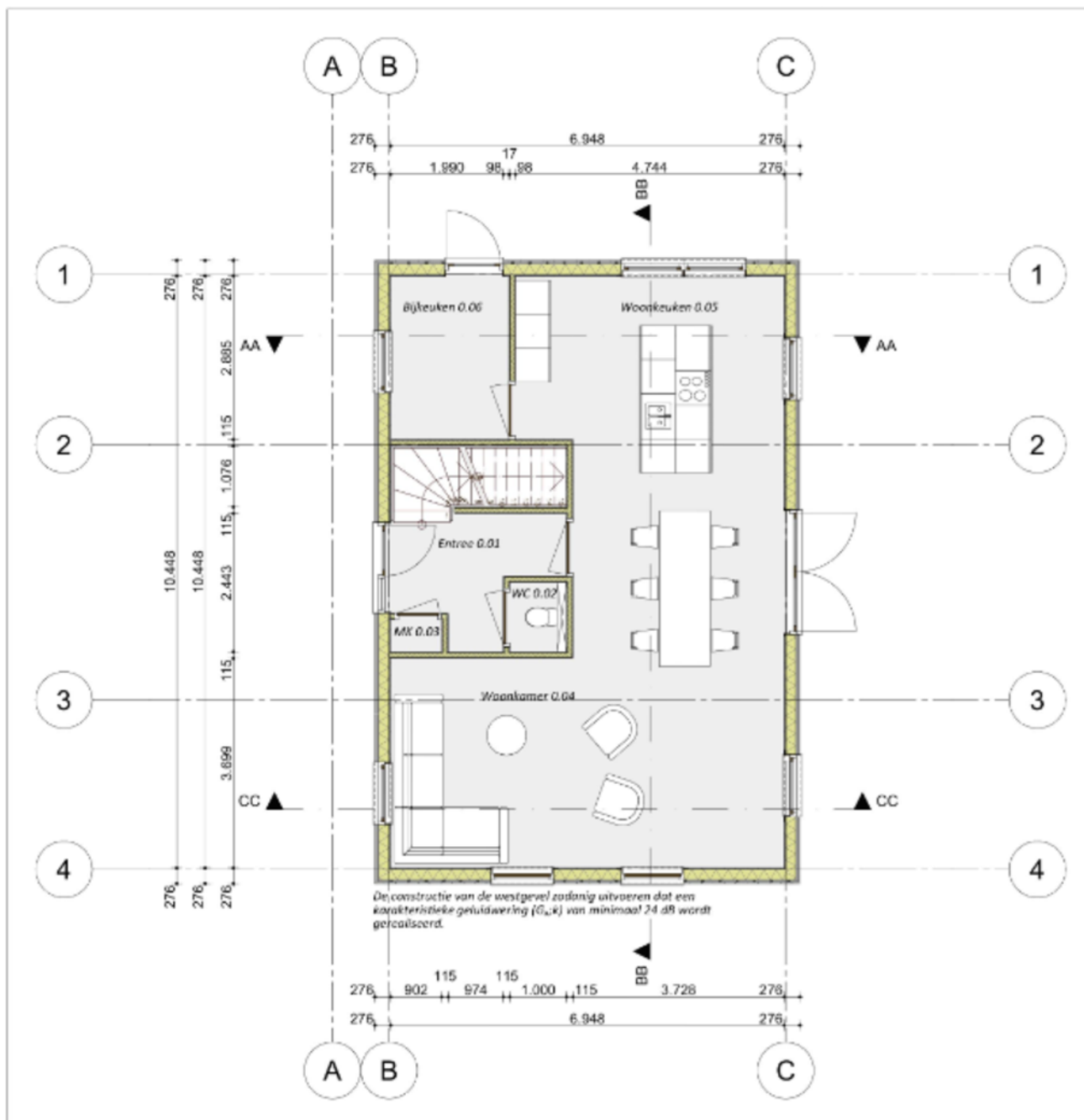
Plattegrond woonhuis
