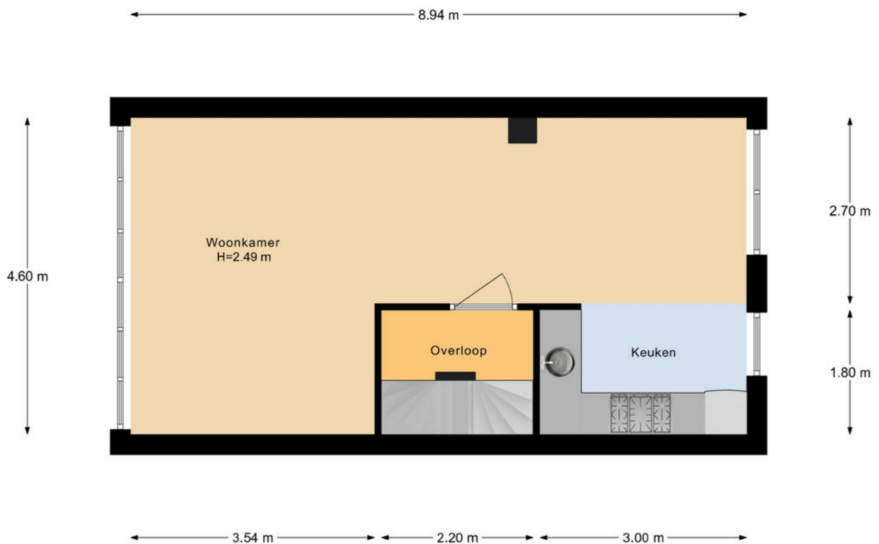
1e Verdieping
