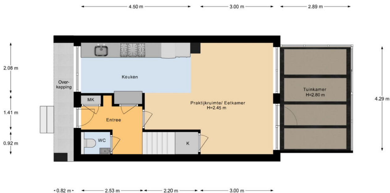
Begane Grond
