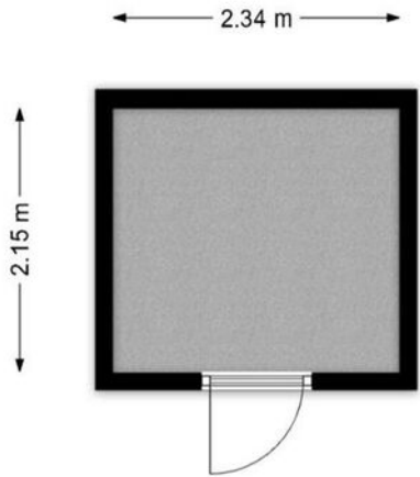
Berging, Louis Armstronglaan 632 te Utrecht, Deze plattegronden zijn opgemaakt voor indicatieve doeleinden. Hieraan kunnen geen rechten worden ontleend.
