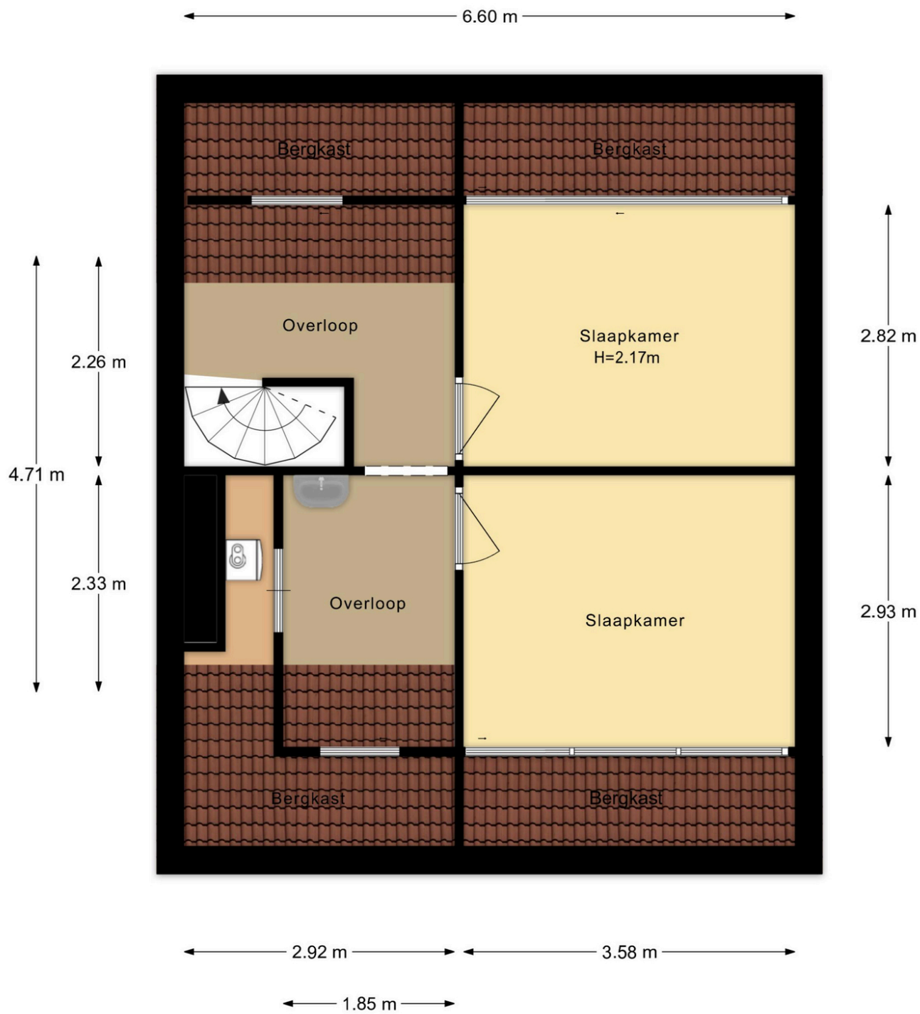
De Ruyterlaan 24 Bennebroek 2e Verdieping
