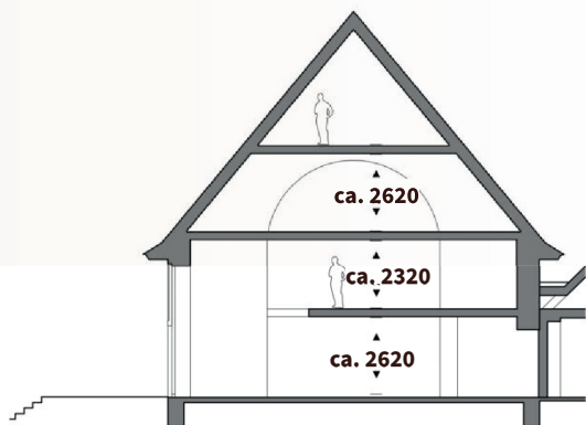
Principedoorssnede (1) woning 5
