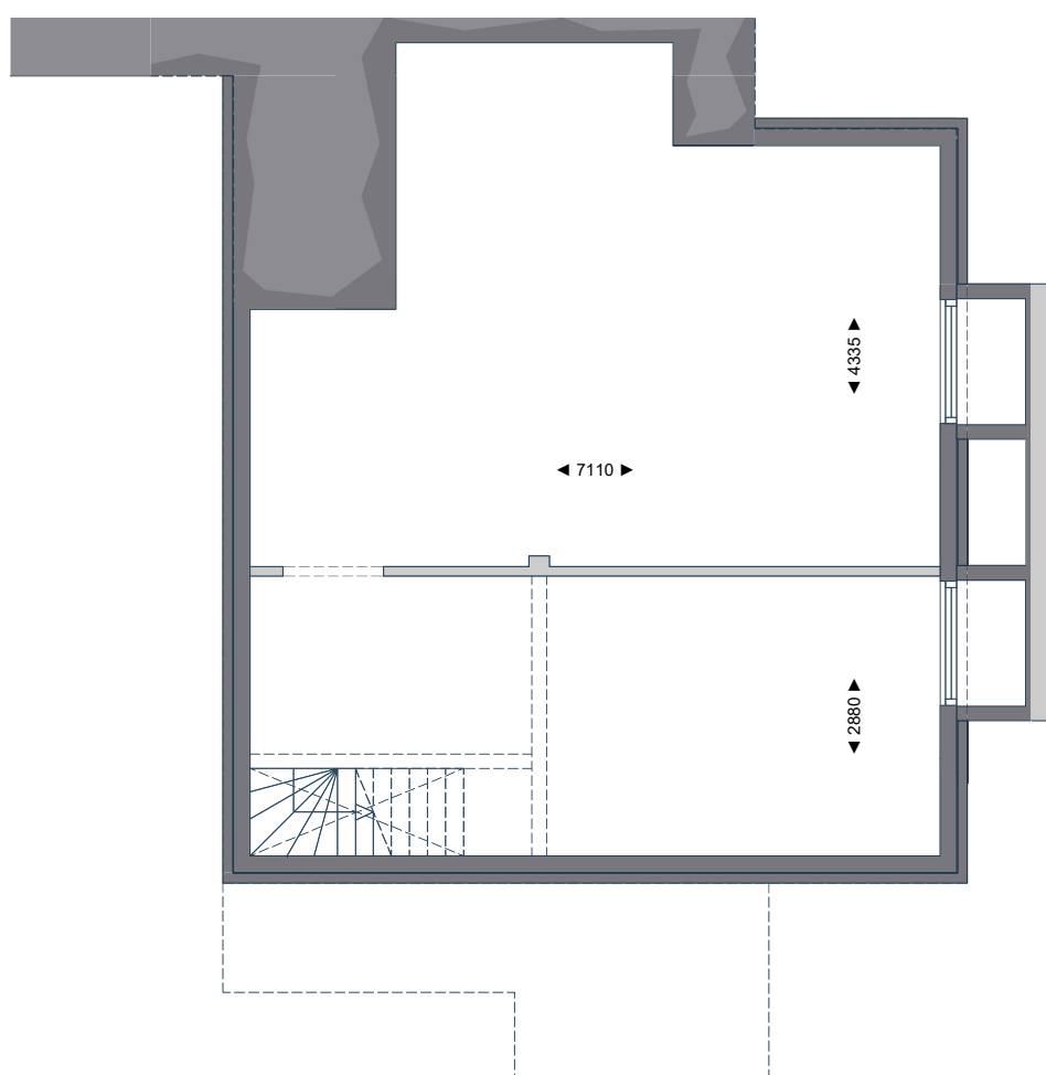
Kelder
