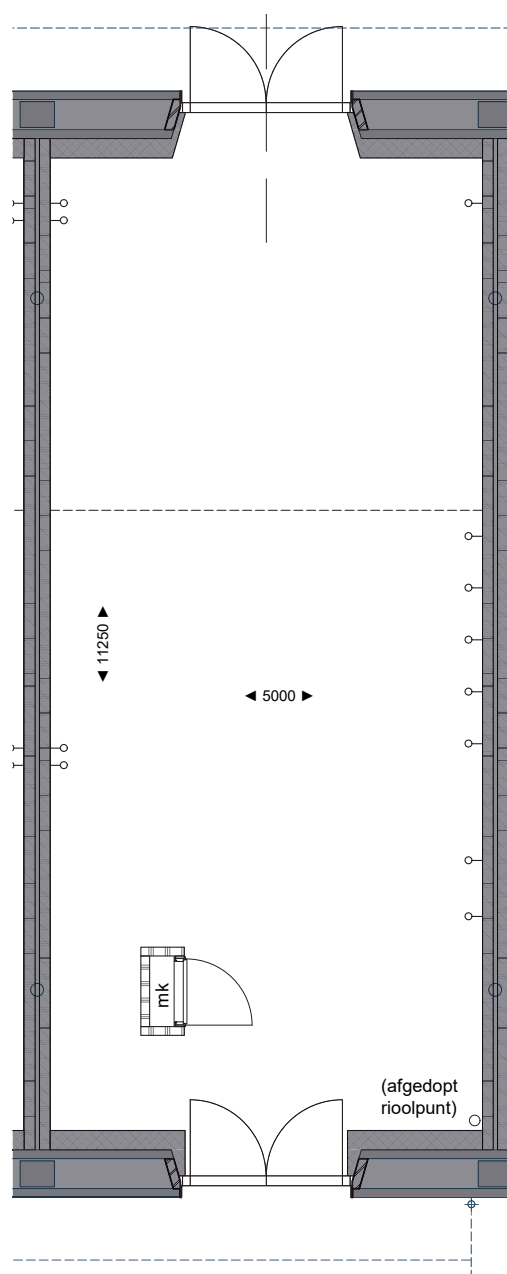
Begane grond
