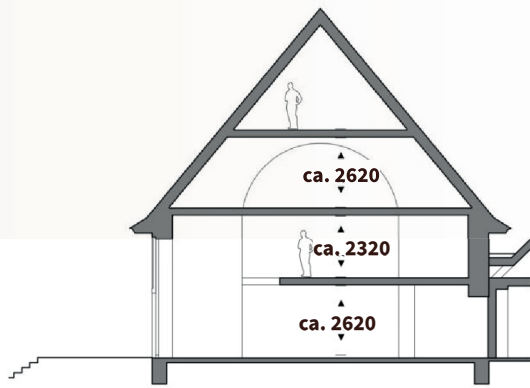
Principedoorsnede (1) woning 5
