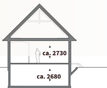
Principedoorsnede woning 6
