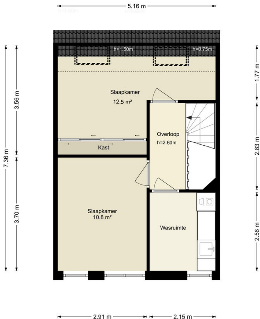
Vuurvlindersingel 104 - Utrecht Tweede Verdieping
