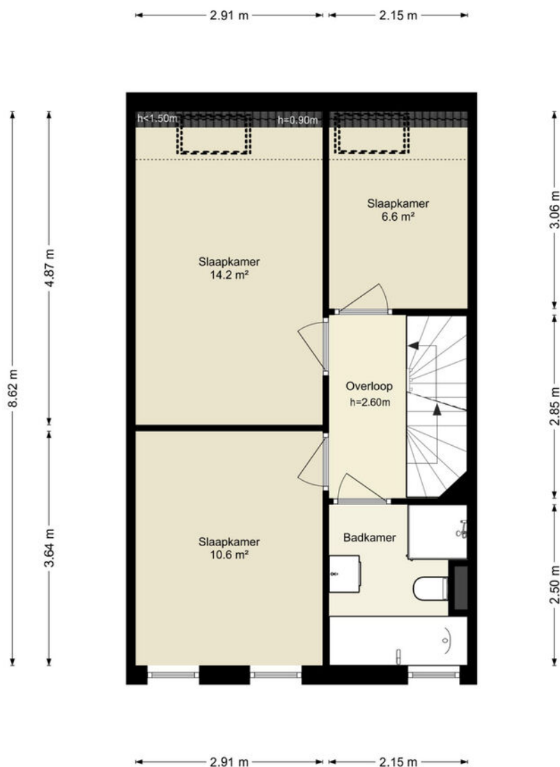
Vuurvlindersingel 104 - Utrecht Eerste Verdieping
