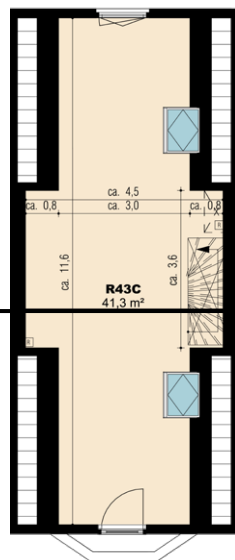
Derde verdieping
