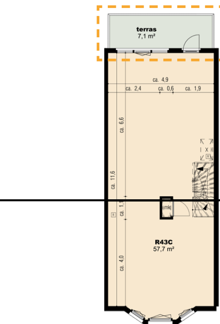
Tweede verdieping
