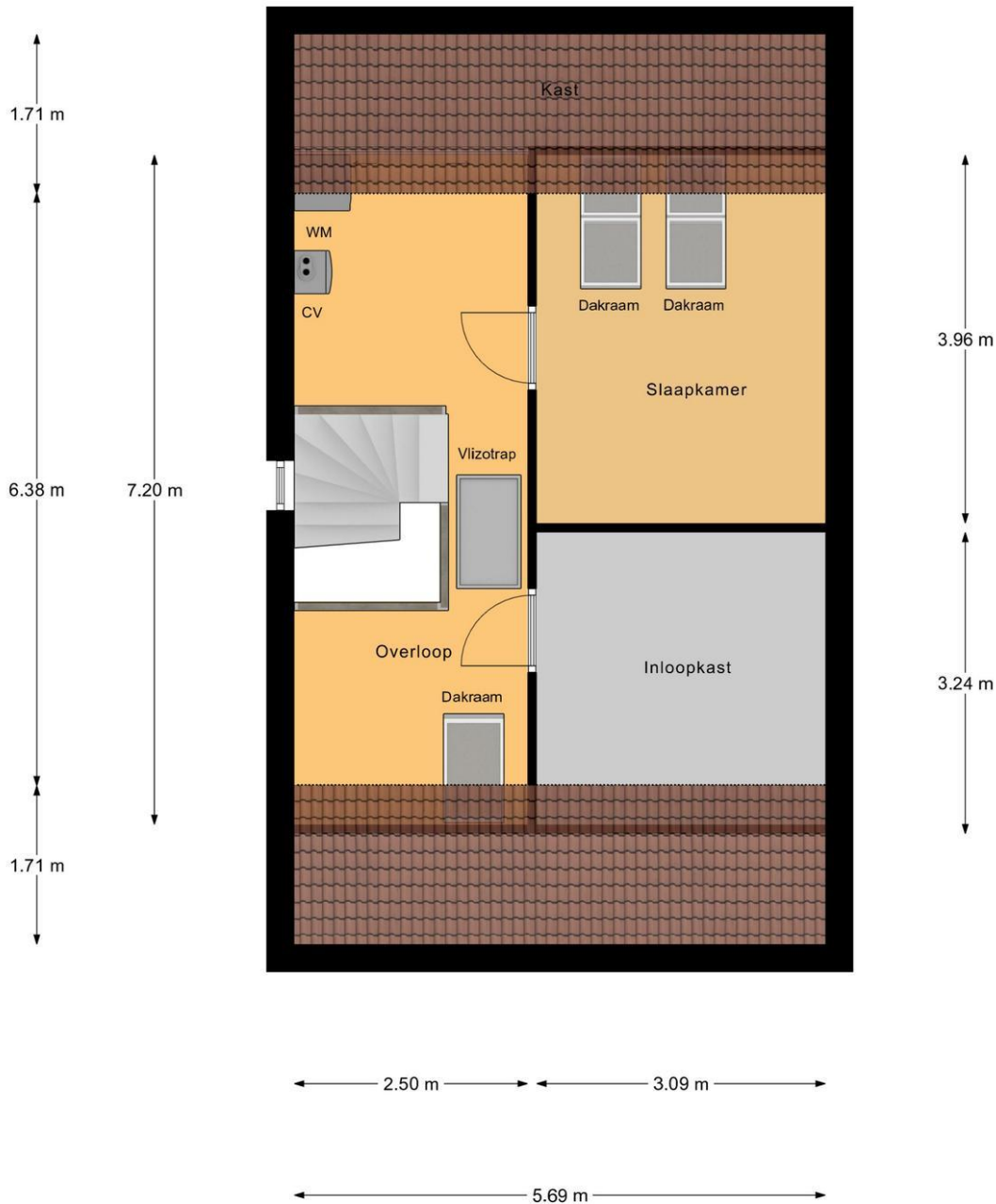
2e Verdieping
