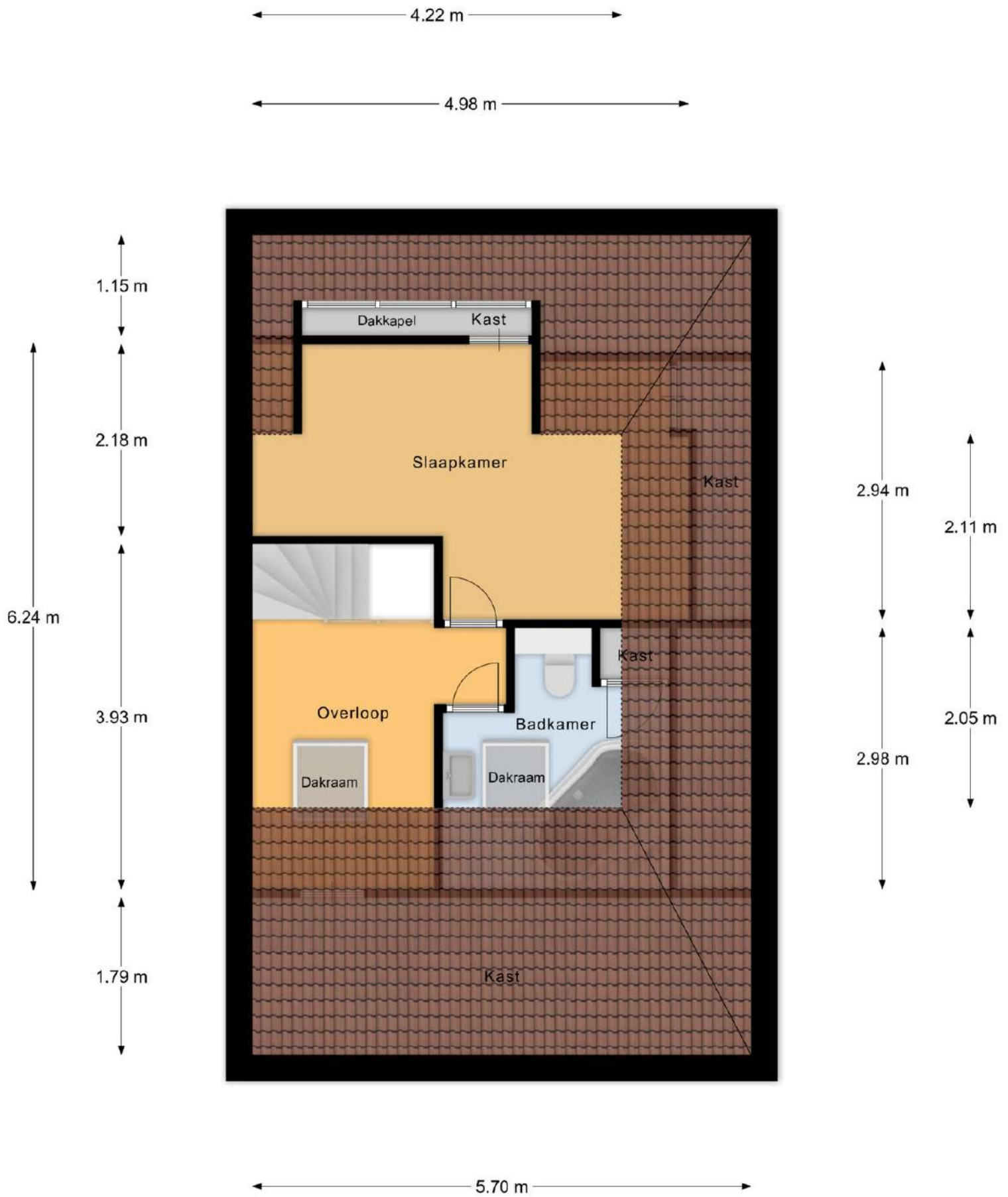
2e Verdieping
