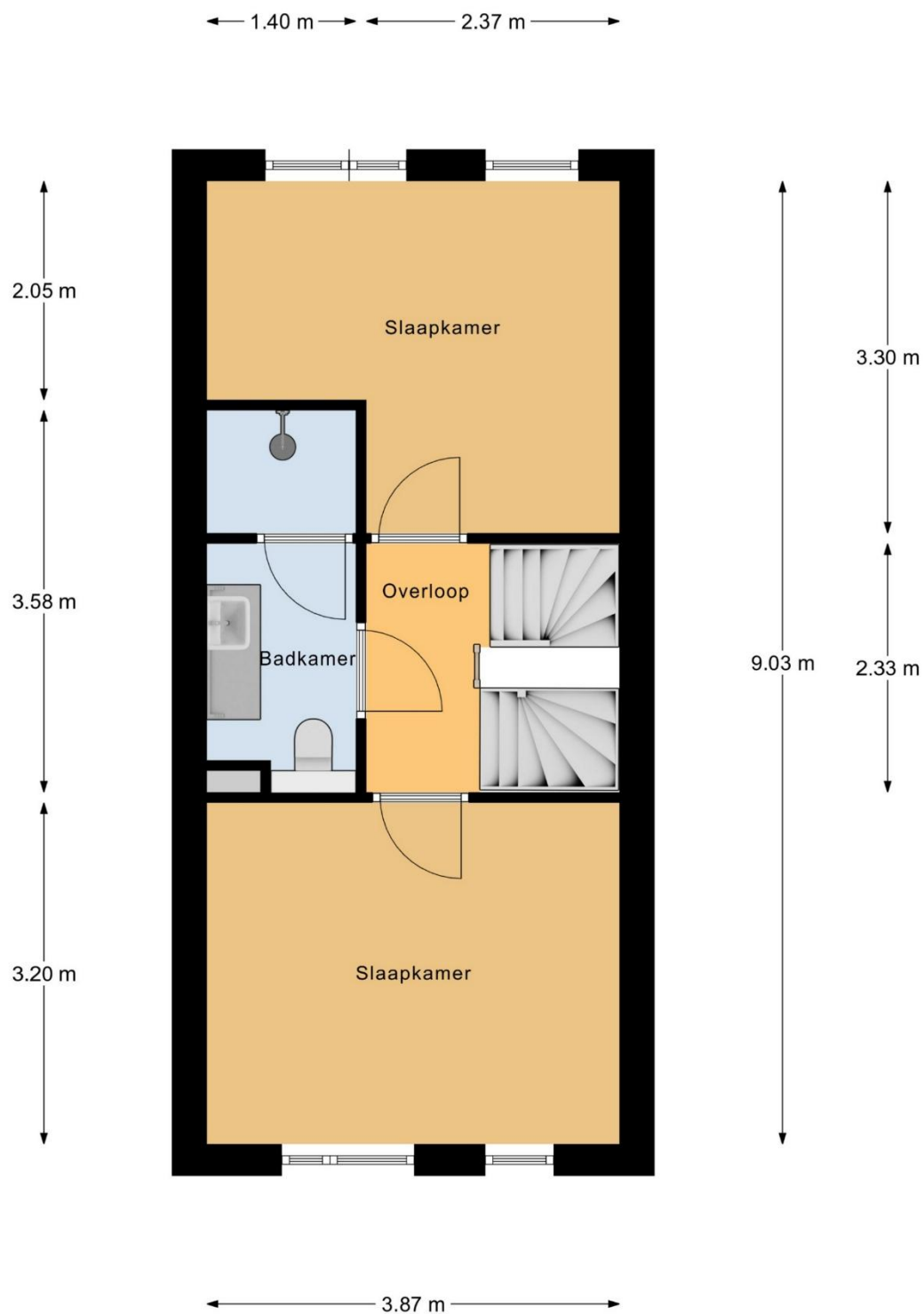
1e Verdieping
