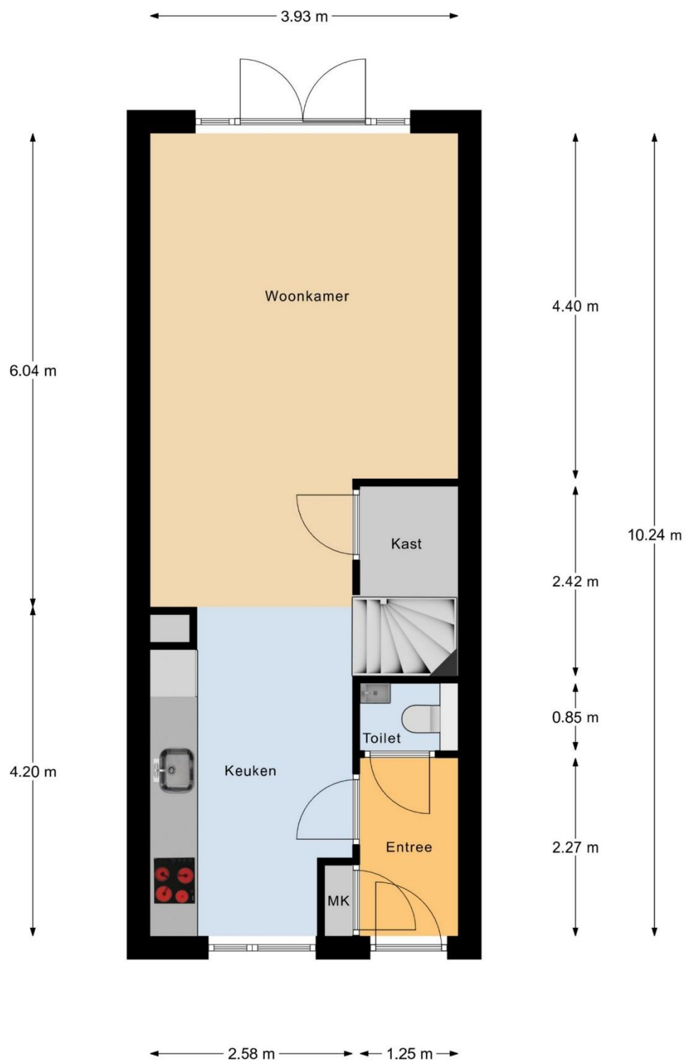
Begane Grond
