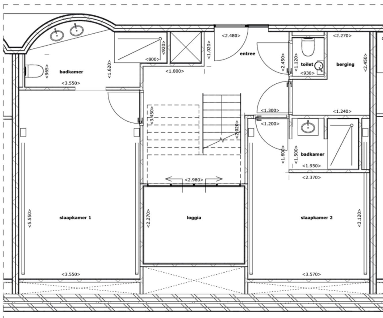
Plattegrond verdieping 03 1:50
