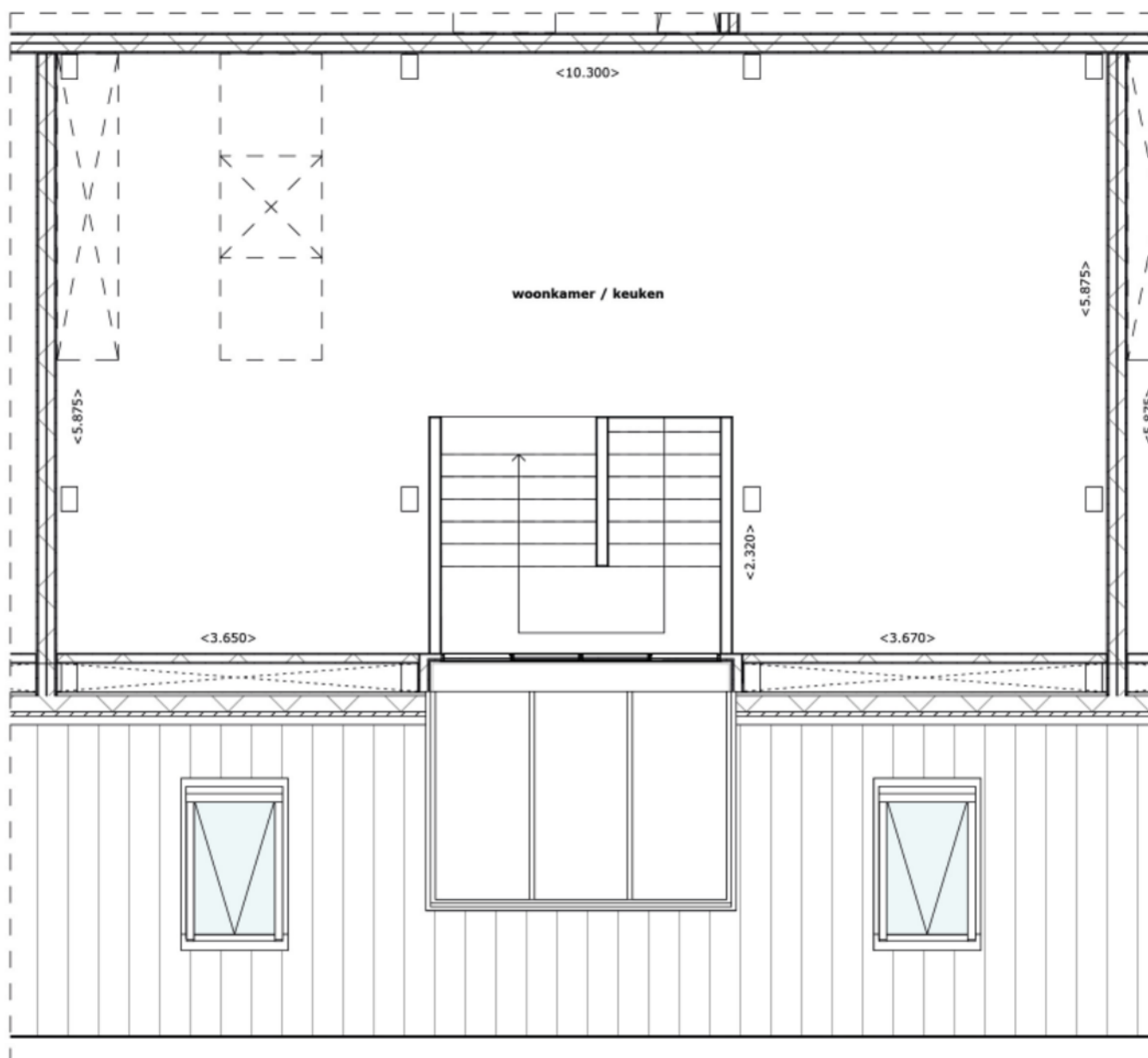
Plattegrond verdieping 04 1:50
