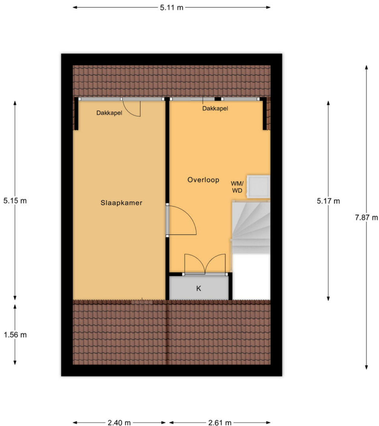
2e Verdieping
