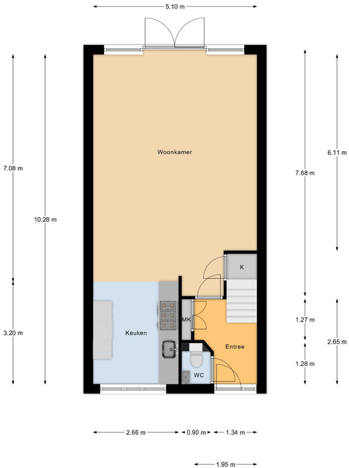
Begane Grond
