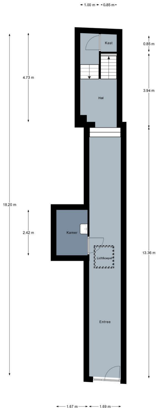
Begane Grond
