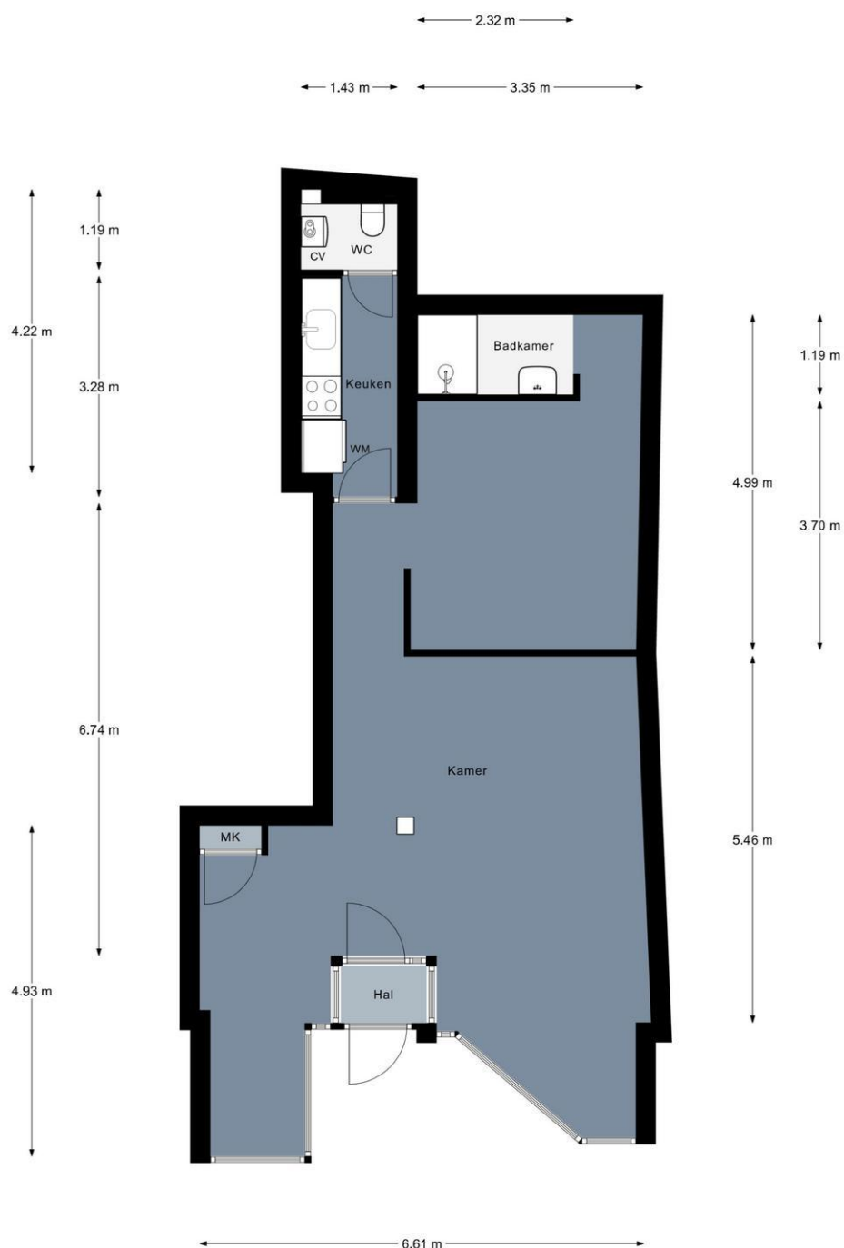
Plattegrond
