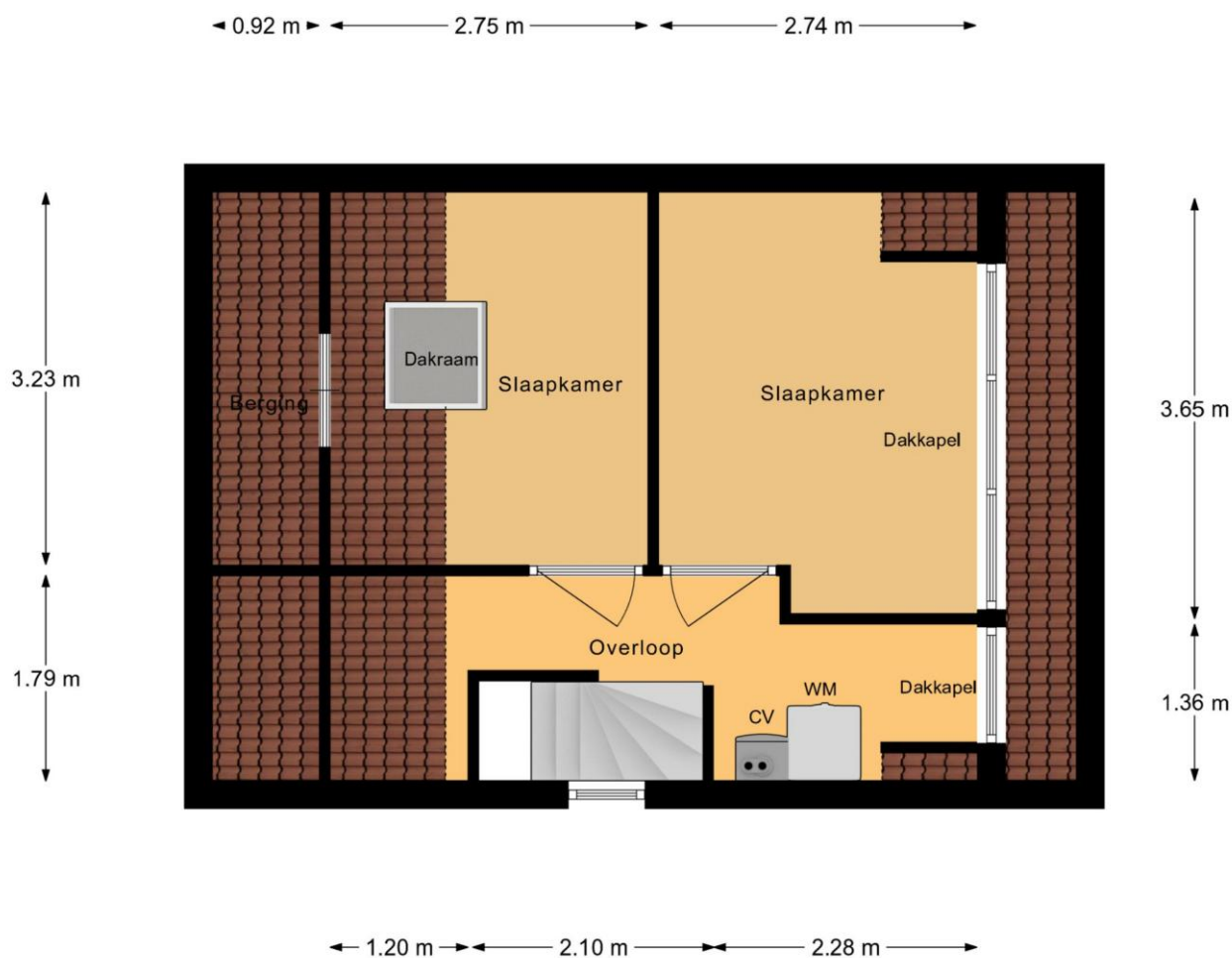
2e Verdieping
