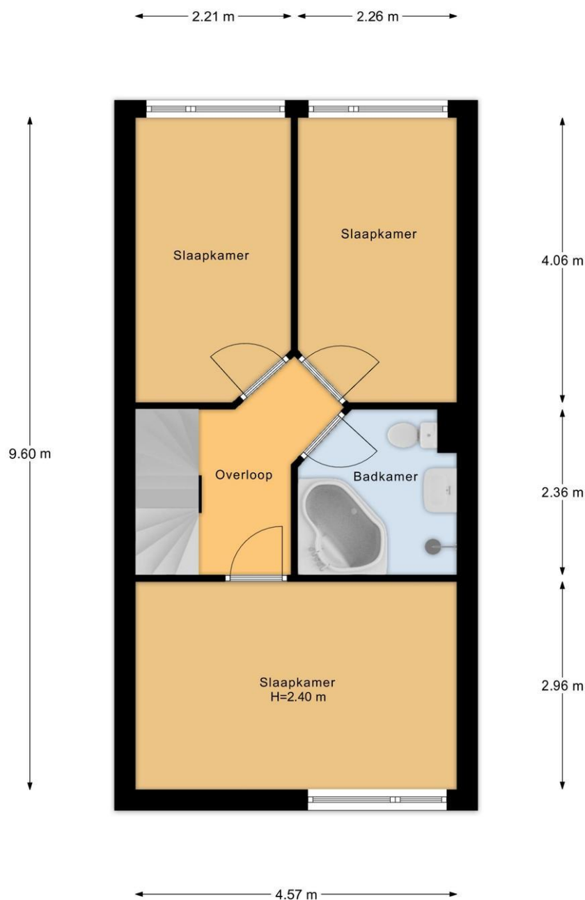
1e Verdieping
