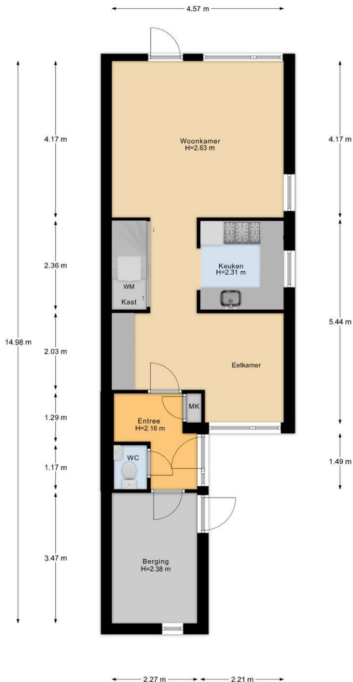
Begane Grond
