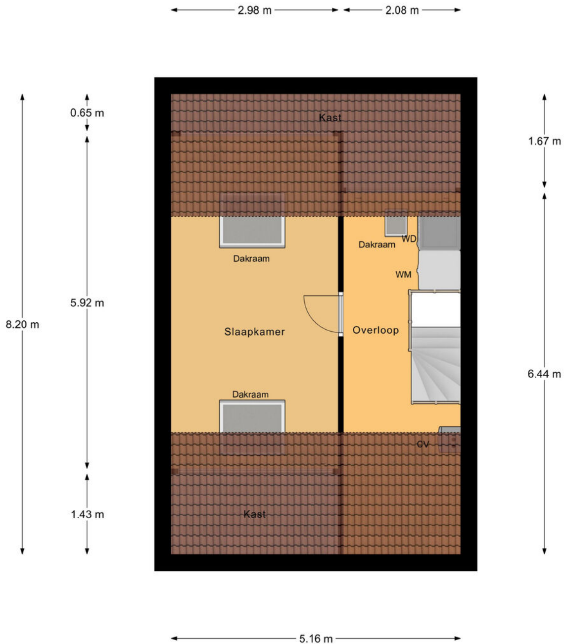
2e Verdieping
