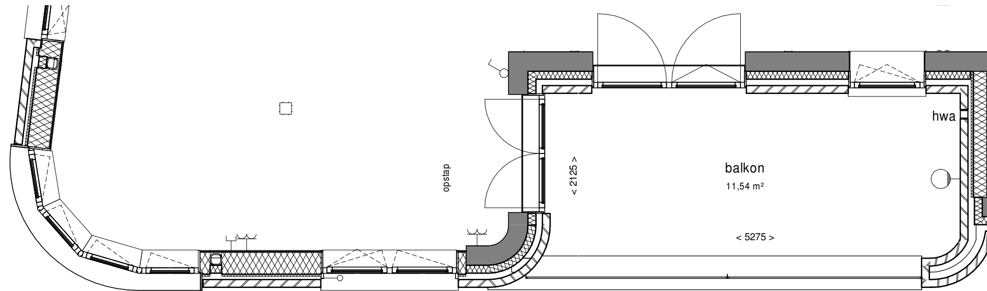
westgevel Bouwnrs.: 03.21/05.16
