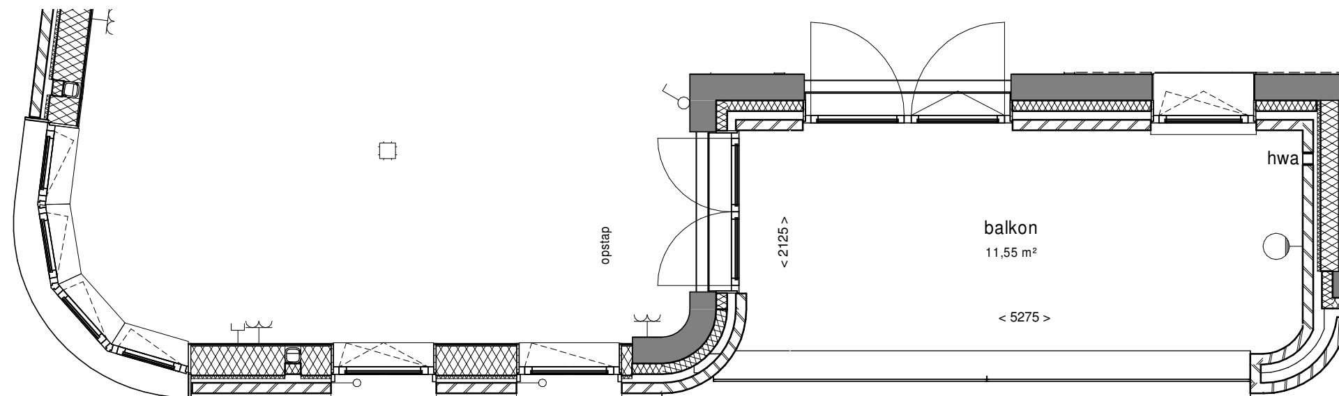
westgevel Bouwnrs.: 04.21/06.10
