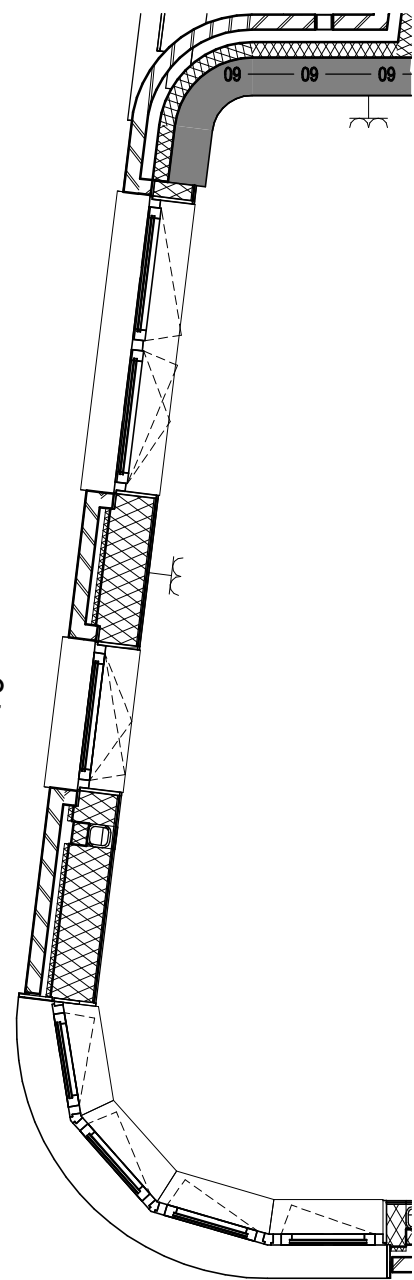
noordgevel Bouwnrs.: 03.21/05.16
